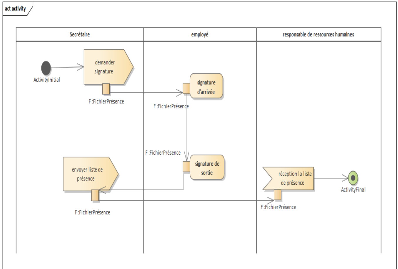
FIGURE 1.4 – Diagramme d'activité du processus métier : gestion de présence
