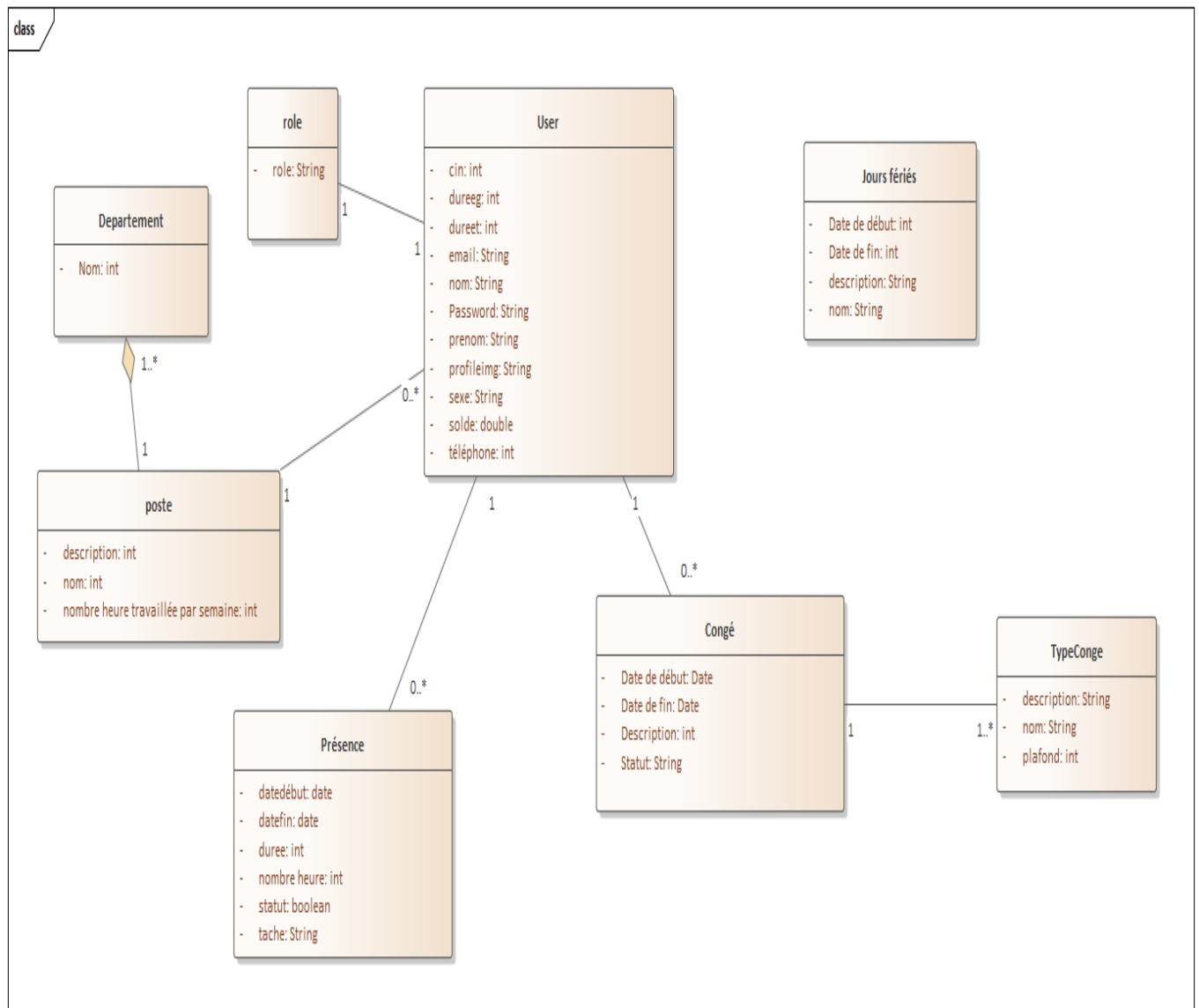
FIGURE 3.24 – Diagramme de classes du domaine
