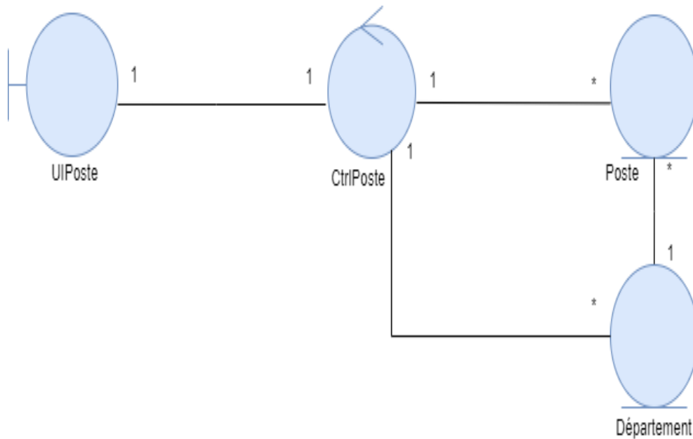
FIGURE 3.13 – Diagramme de classes participantes du scénario «Ajouter un nouveau poste»
