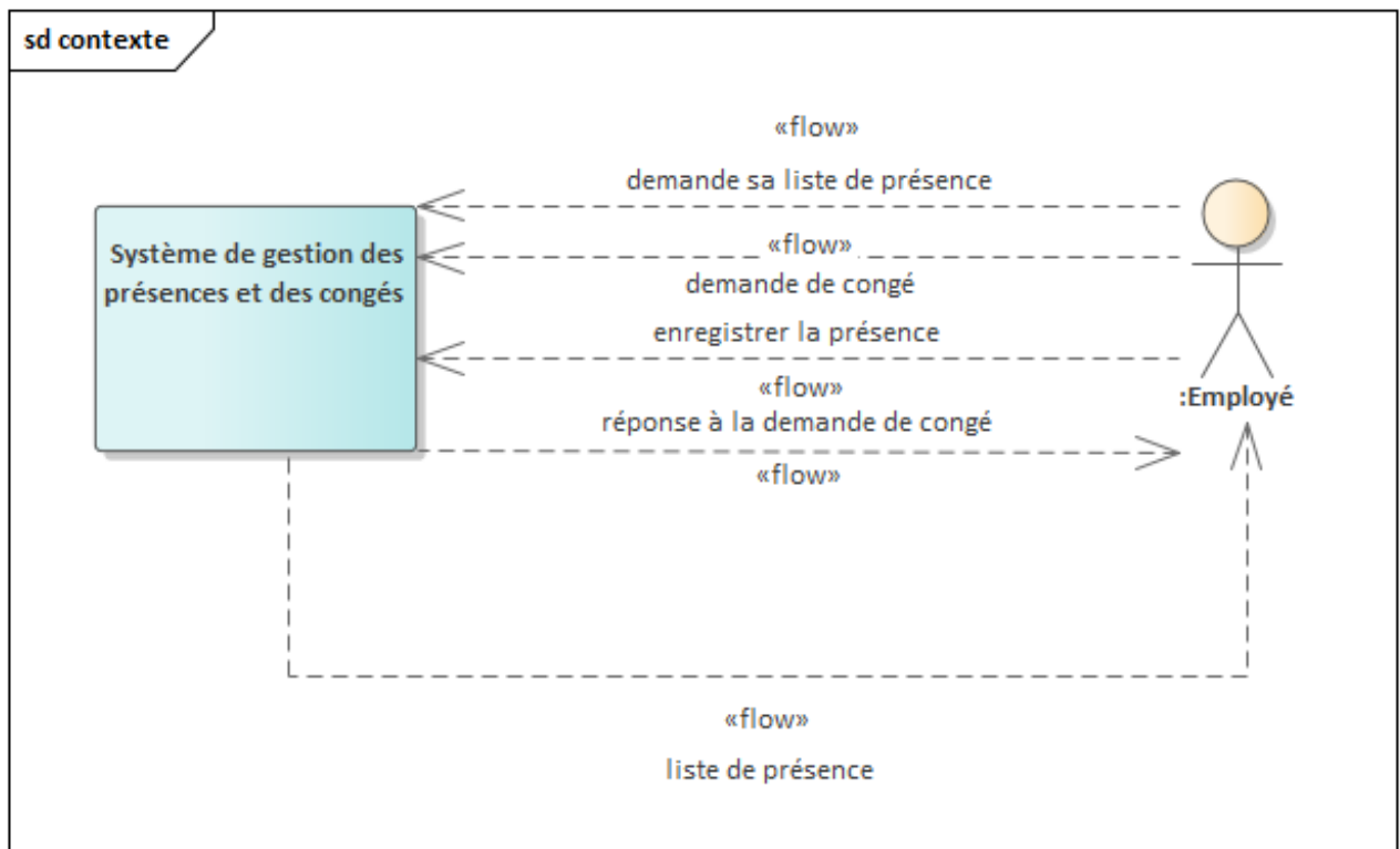
FIGURE 1.1 – Diagramme de contexte métier
