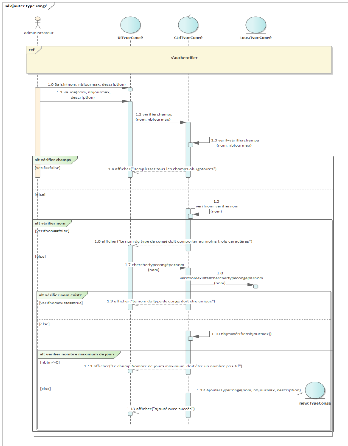
FIGURE 3.14 – Diagramme de séquence du scénario «Ajouter un nouveau Type De Congé»
