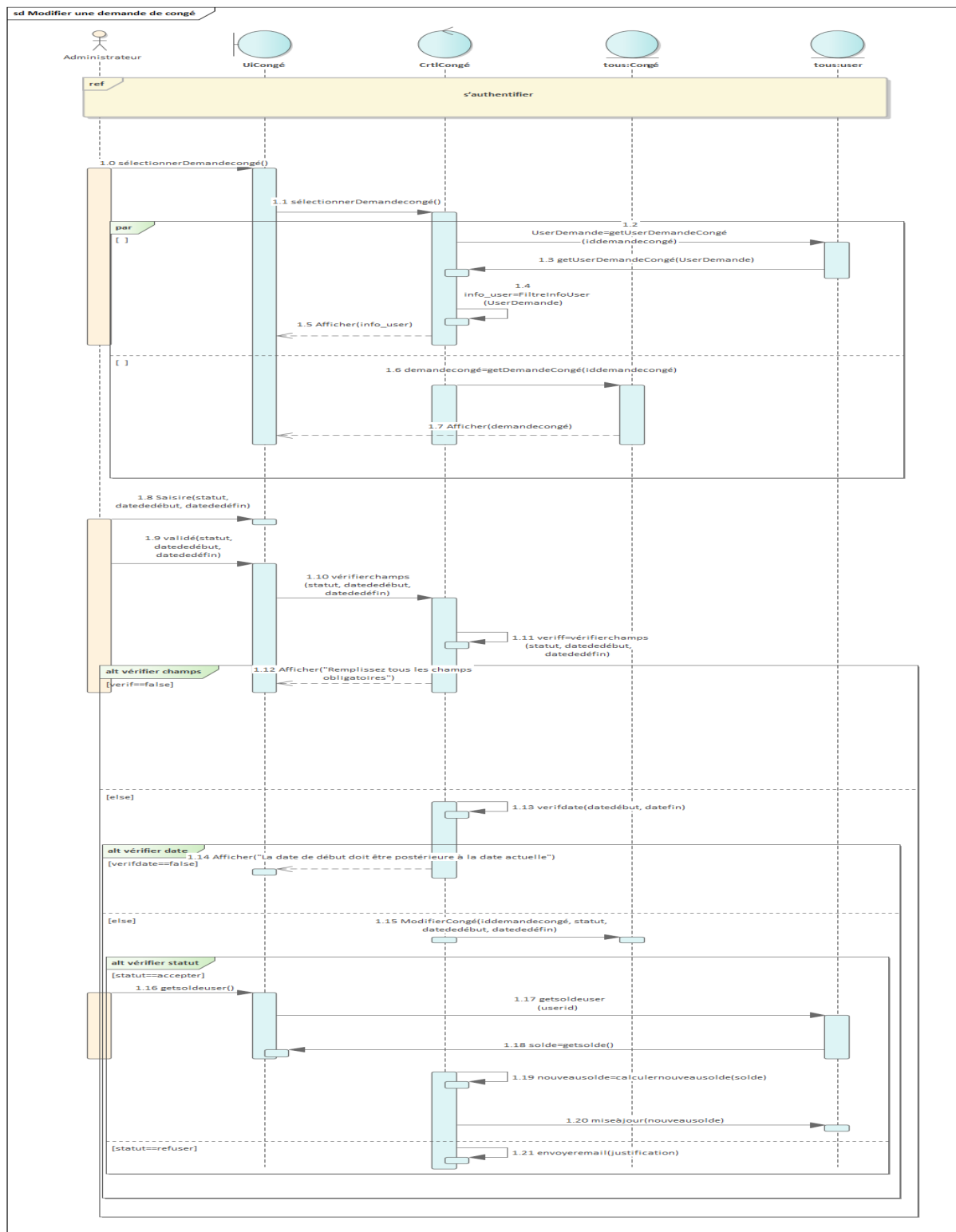
FIGURE 3.22 – Diagramme de séquence du scénario «Modifier une demande de congé»
