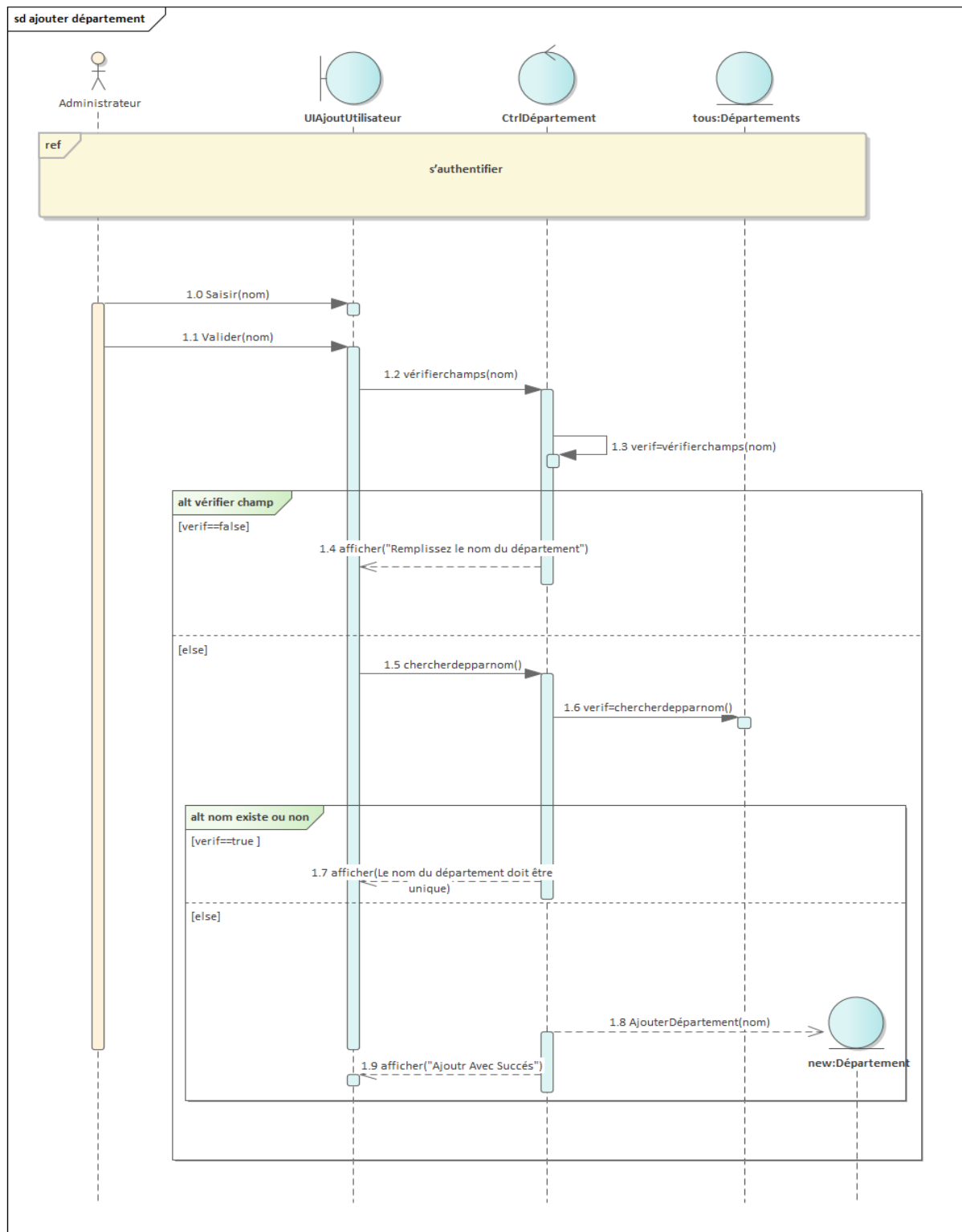
FIGURE 3.10 – Diagramme de séquence du scénario « Ajouter un nouveau département »
