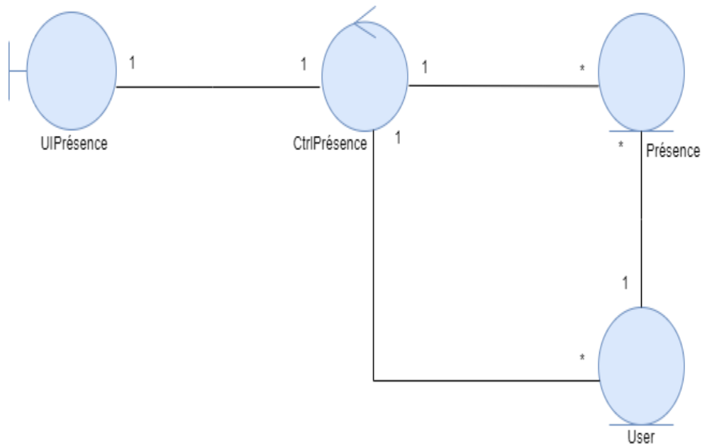
FIGURE 3.17 – Diagramme de classes participantes du scénario «modifier présence»
