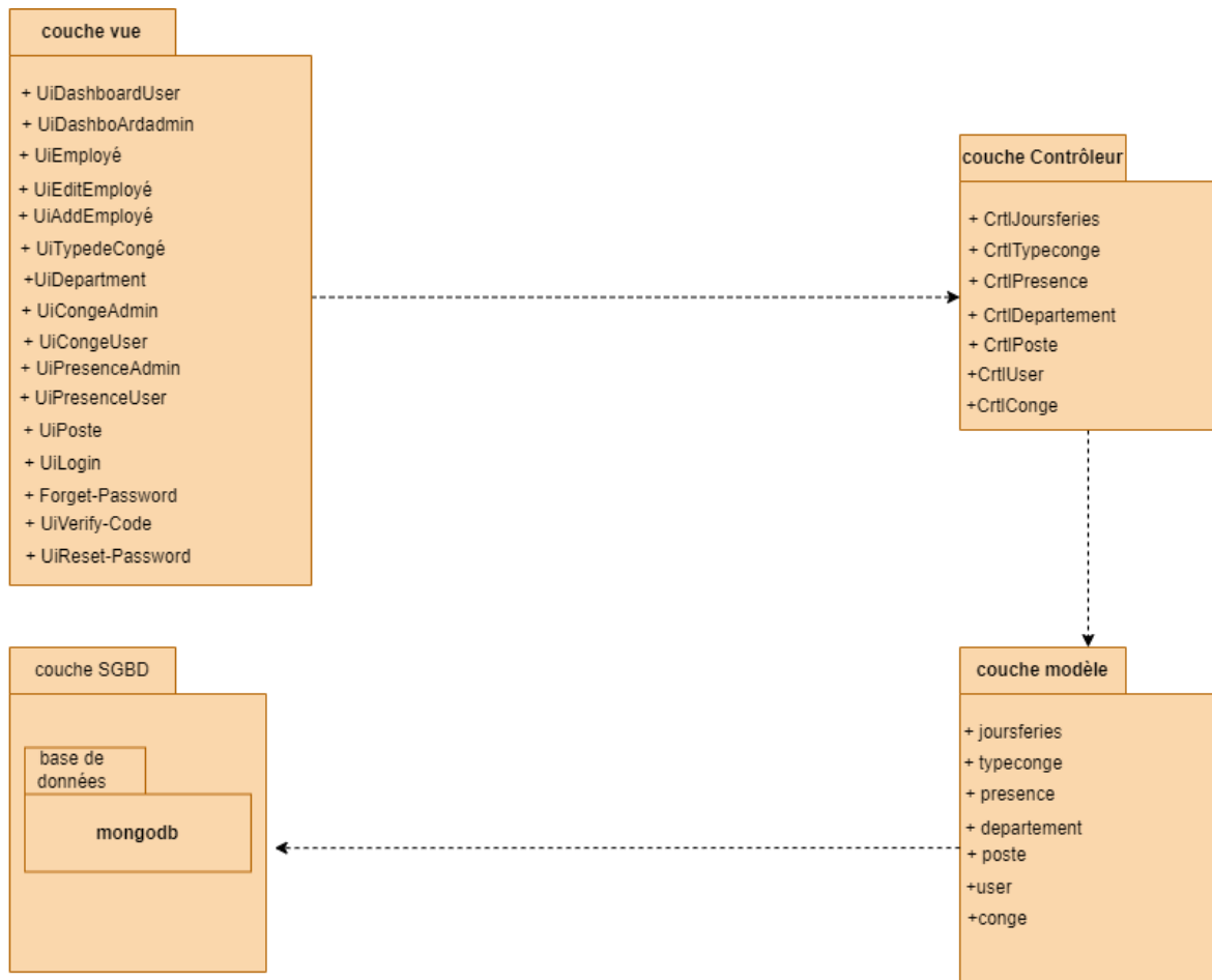
FIGURE 3.25 – Diagramme de paquetage
