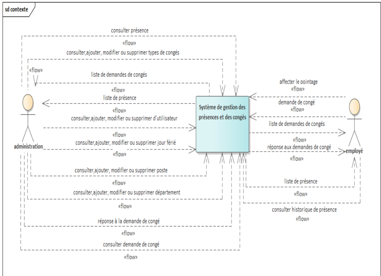
FIGURE 2.2 – Modèle de contexte du système informatisé
