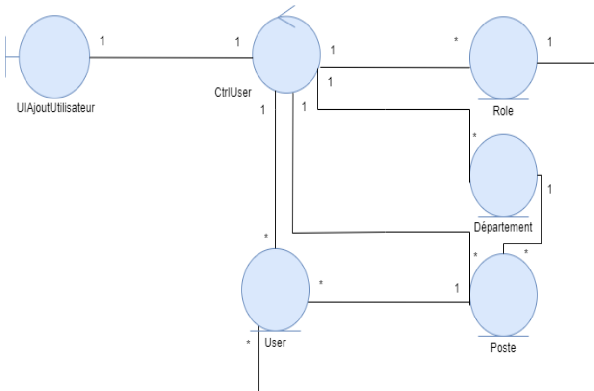
FIGURE 3.7 – Diagramme de classes participantes du scénario «Ajouter un nouvel utilisateur»
