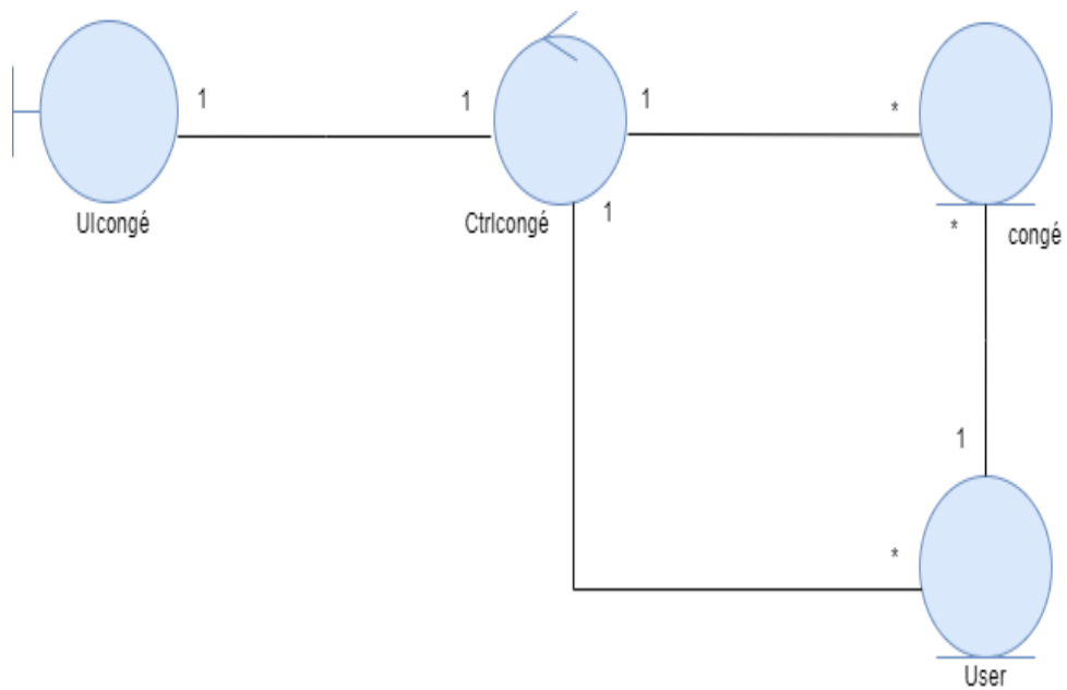
FIGURE 3.23 – Diagramme de classes participantes du scénario «Modifier une demande de congé»
