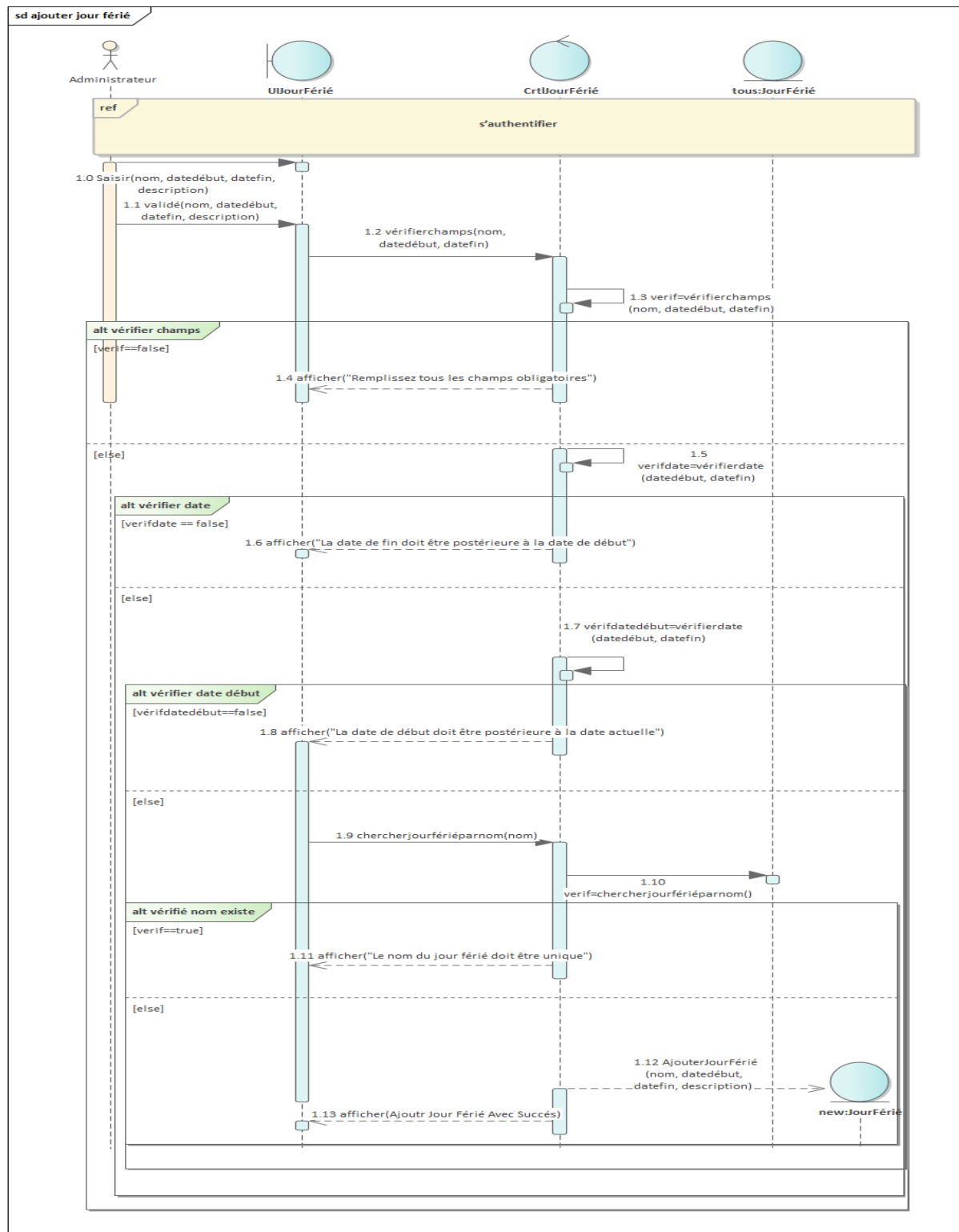
FIGURE 3.8 – Diagramme de séquence du scénario « Ajouter un nouveau jour férié »
