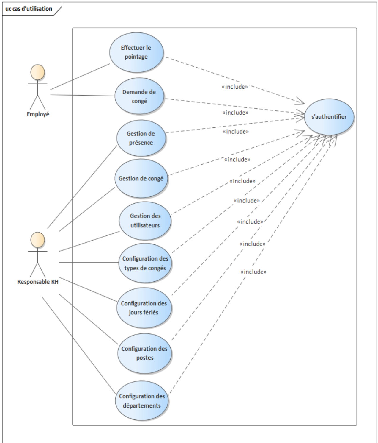
FIGURE 2.3 – Diagramme de cas d'utilisation du système informatisé
