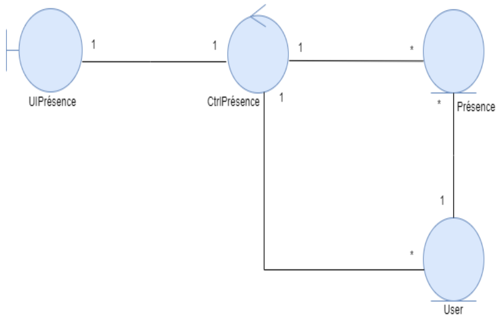
FIGURE 3.19 – Diagramme de classes participantes du scénario «Ajouter une présence»
