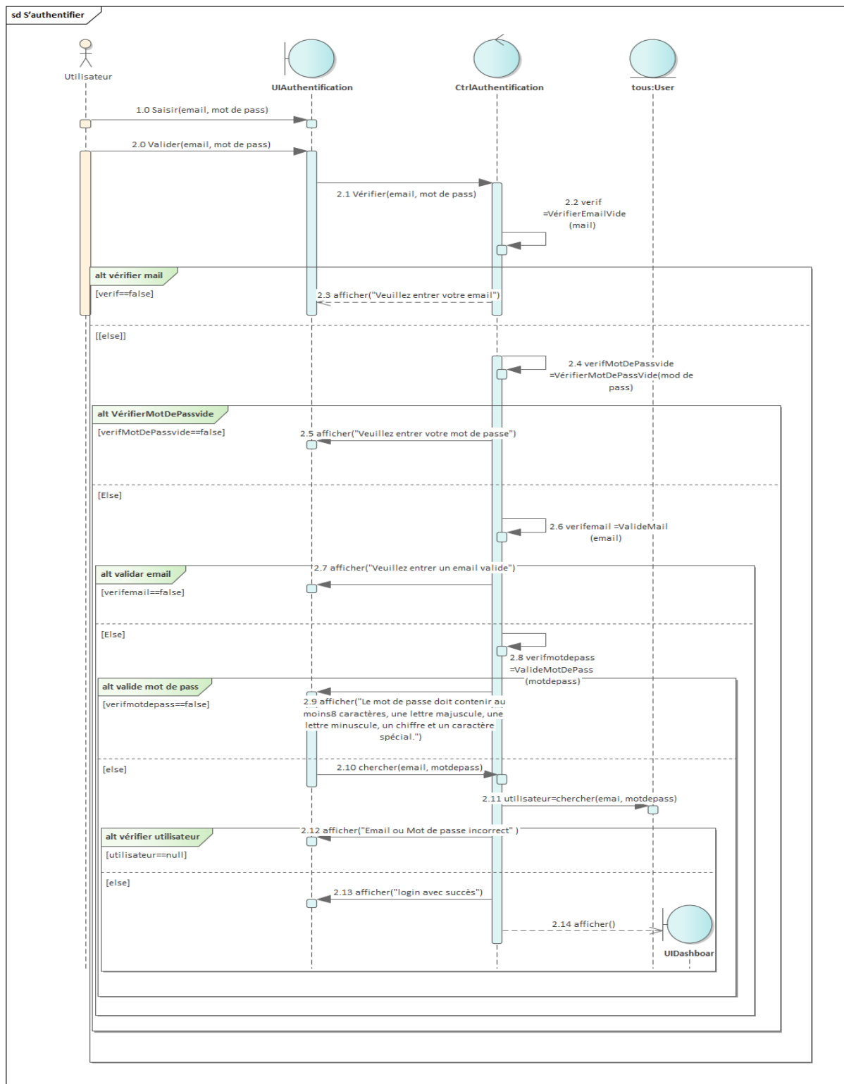
FIGURE 3.4 – Diagramme de séquence du scénario «S'authentifier»
