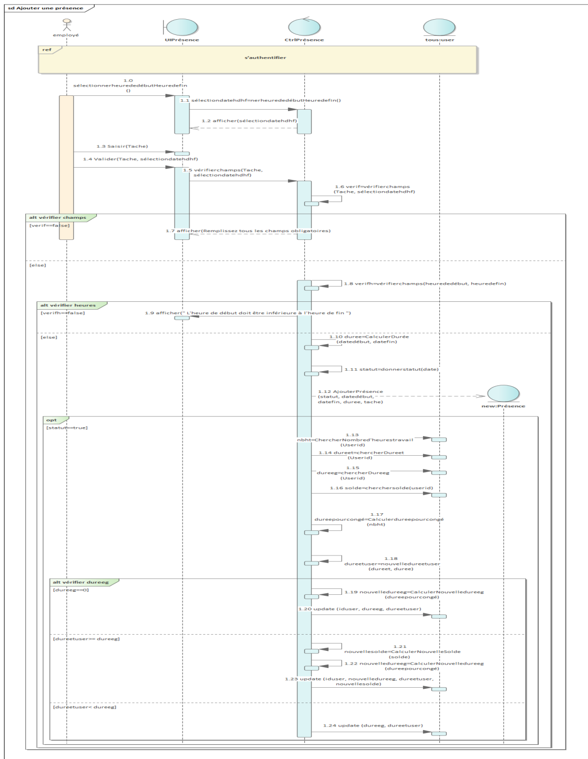
FIGURE 3.18 – Diagramme de séquence du scénario «Ajouter une présence»
