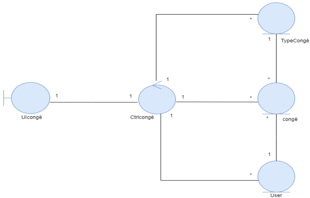
FIGURE 3.21 – Diagramme de classes participantes du scénario «Ajouter une demande de congé»
