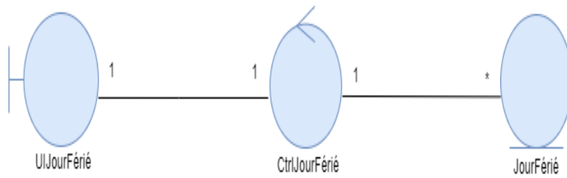
FIGURE 3.9 – Diagramme de classes participantes du scénario «Ajouter un nouveau jour férié»
