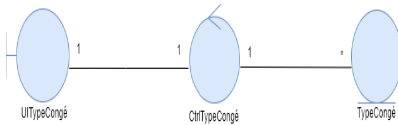
FIGURE 3.15 – Diagramme de classes participantes du scénario «Ajouter un nouveau Type De Congé»
