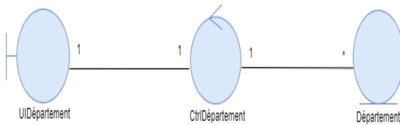
FIGURE 3.11 – Diagramme de classes participantes du scénario «Ajouter un nouveau département»
