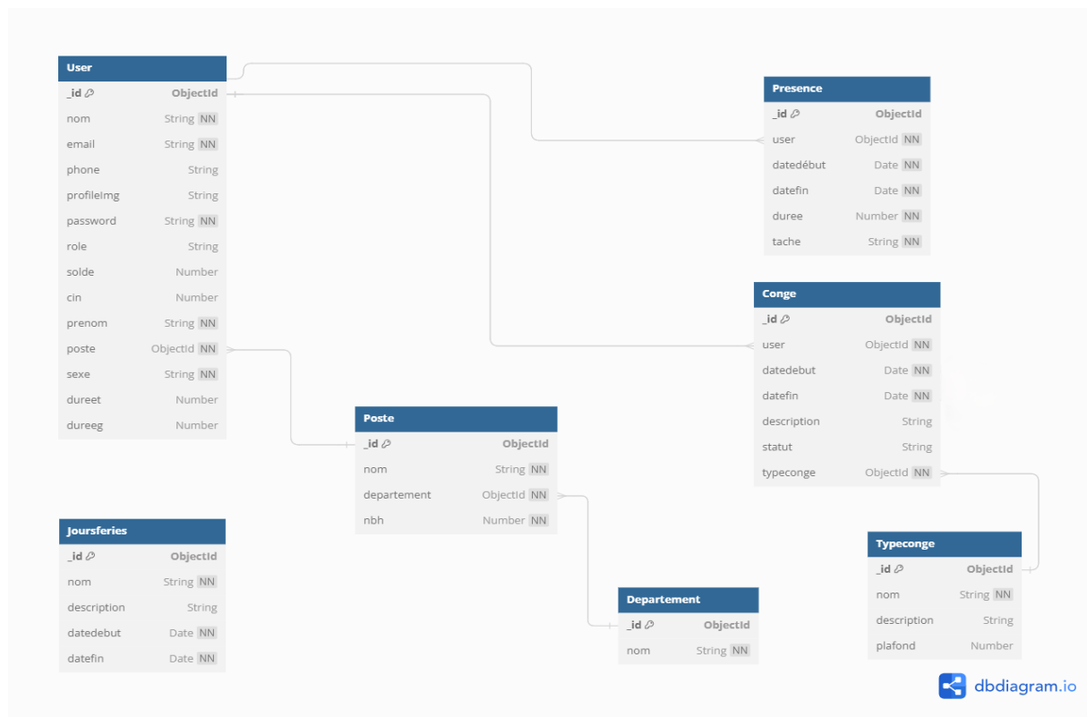
FIGURE 3.26 – Schéma physique de la base de données.
