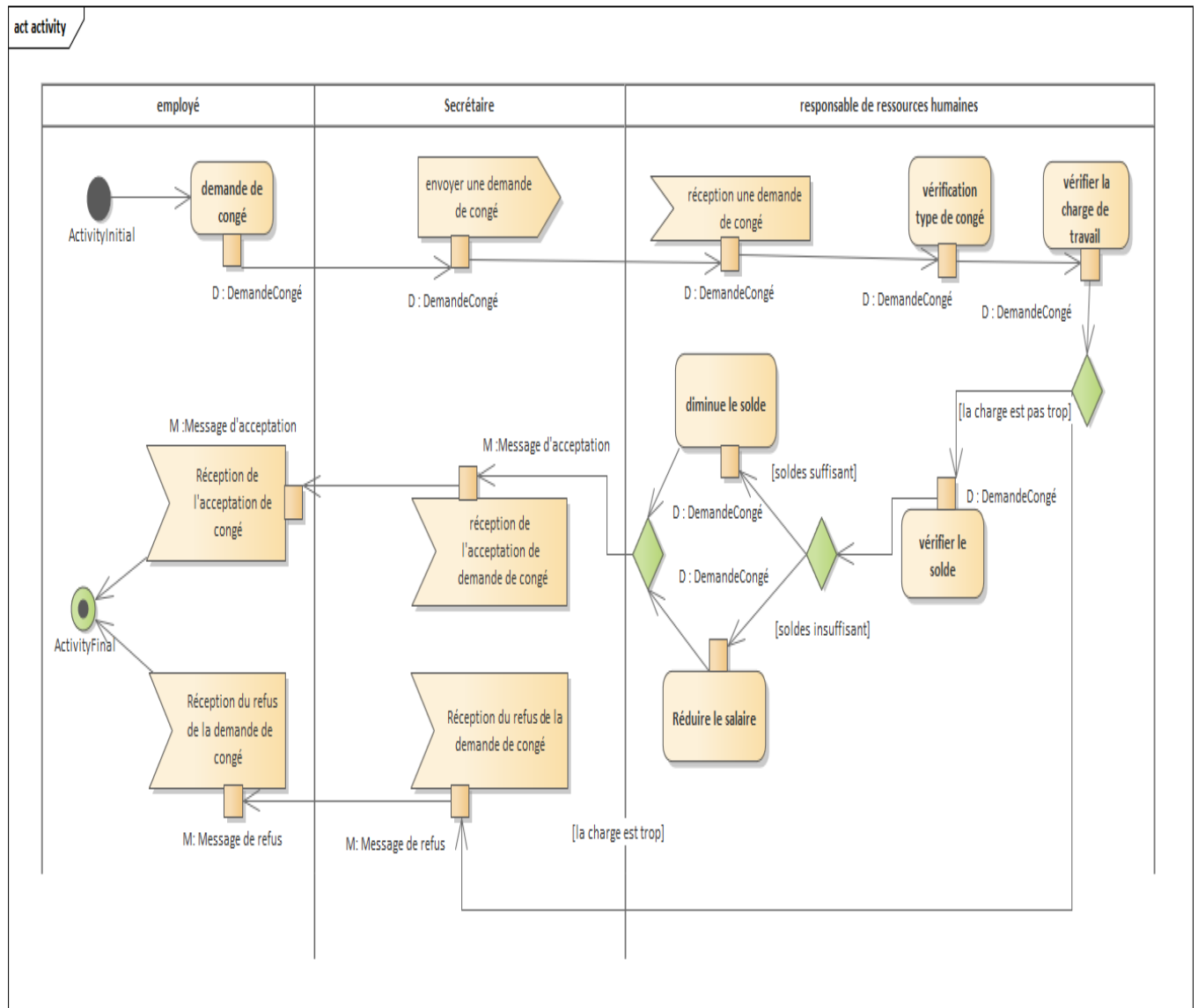
FIGURE 1.5 – Diagramme d’activité du processus métier : gestion de congé
