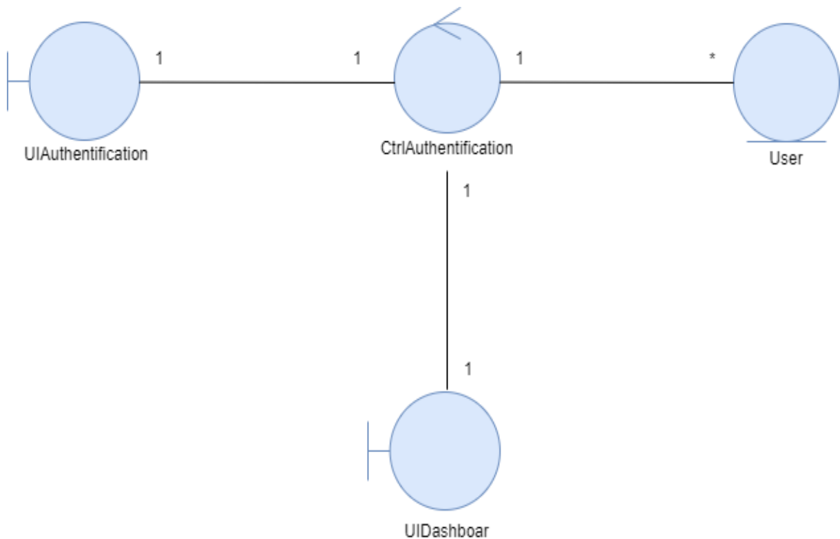
FIGURE 3.5 – Diagramme de classes participantes du scénario «S'authentifier»
