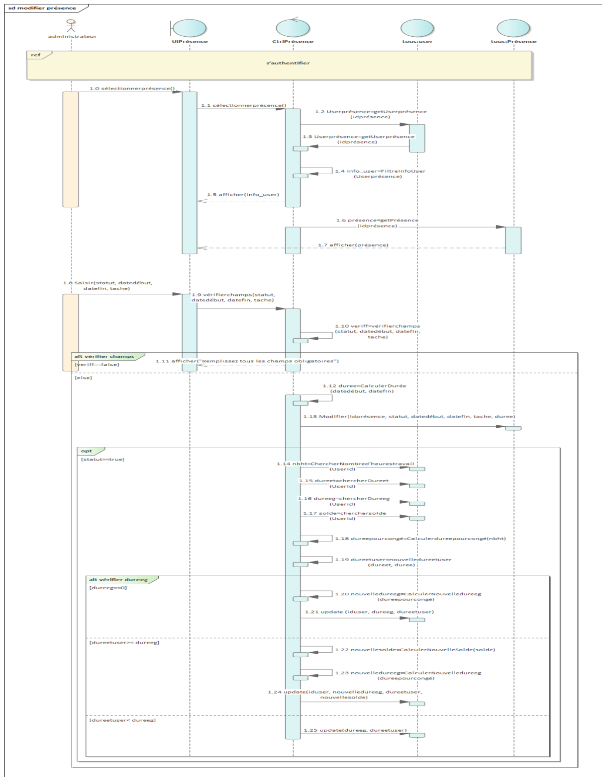
FIGURE 3.16 – Diagramme de séquence du scénario «modifier présence»
