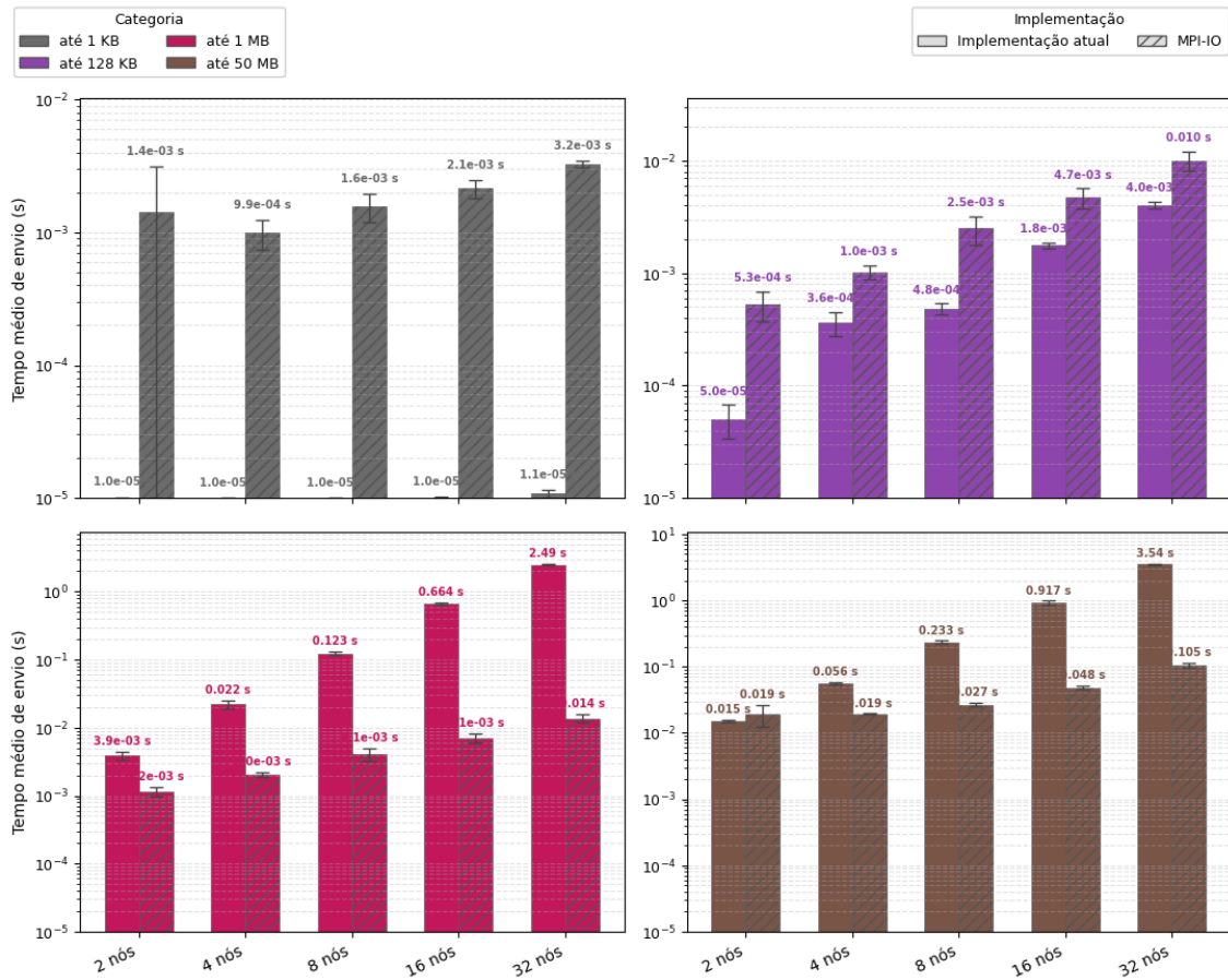
Figura 4.7: Tempo médio de bloqueio das operações de envio em função do tamanho dos blocos de dados no Experimento AWS (escala logarítmica).
