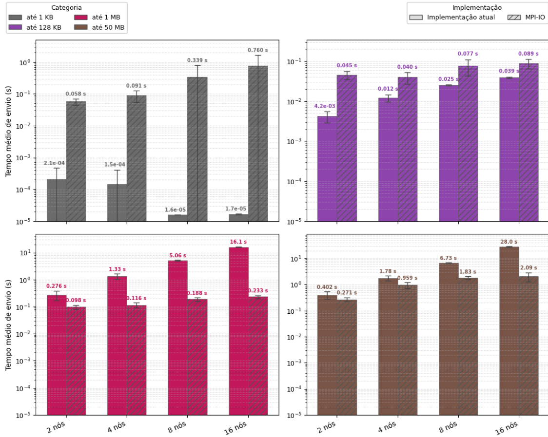
Figura 4.4: Tempo médio de bloqueio das operações de envio por tamanho de bloco de dados nas implementações atual e MPI-IO no Experimento SDumont (escala logarítmica).
