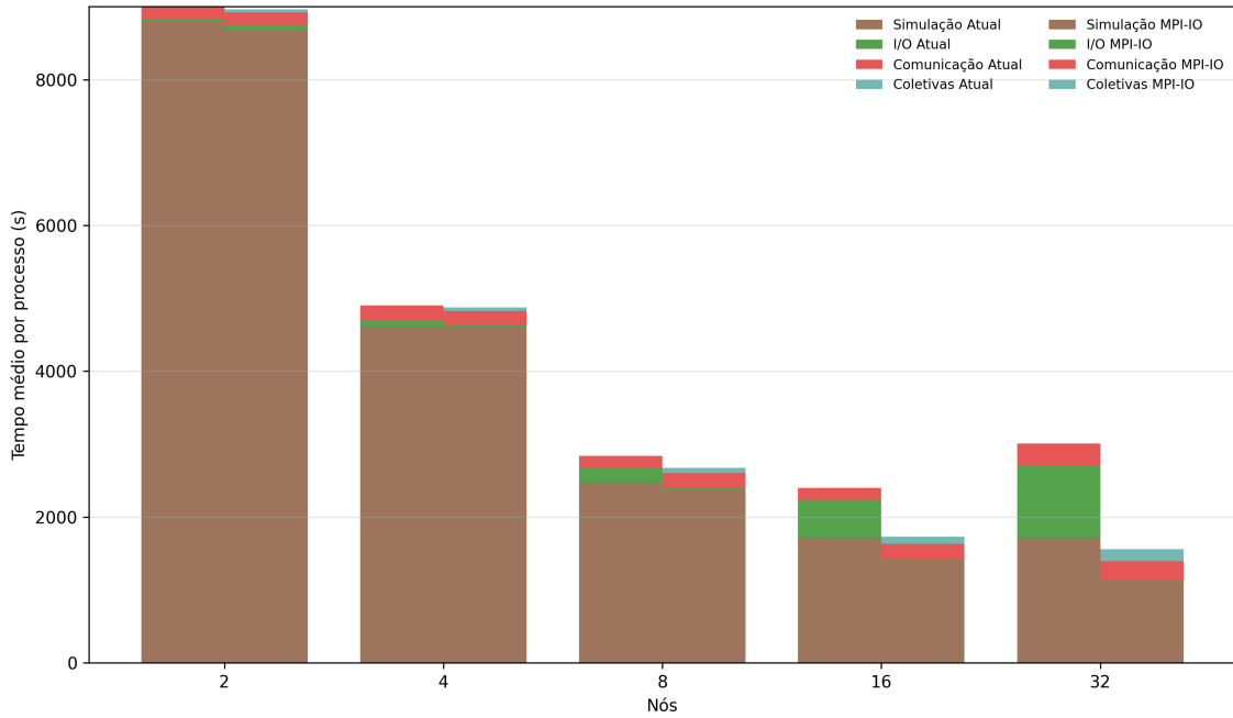
Figura 4.6: Tempo de execução no Experimento AWS.
