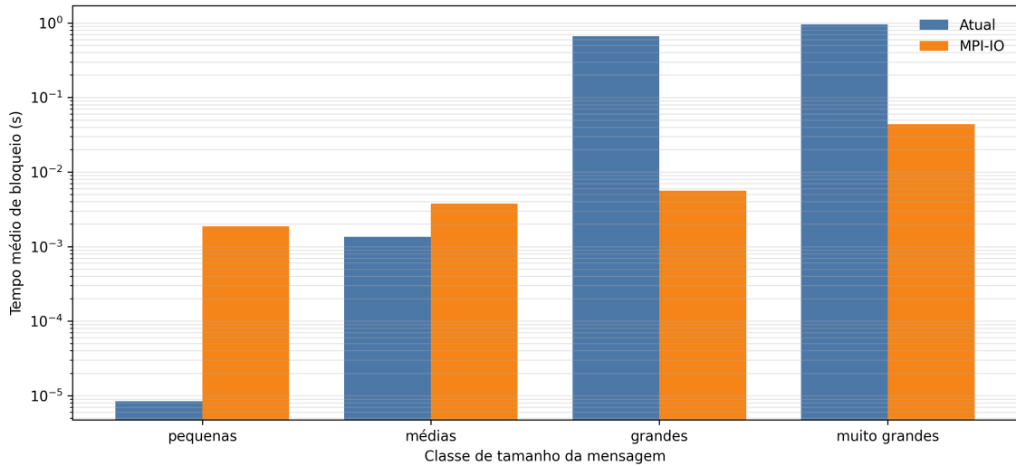
Figura 4.7: Tempo médio de bloqueio das operações de envio em função do tamanho das mensagens no Experimento AWS (escala logarítmica).
