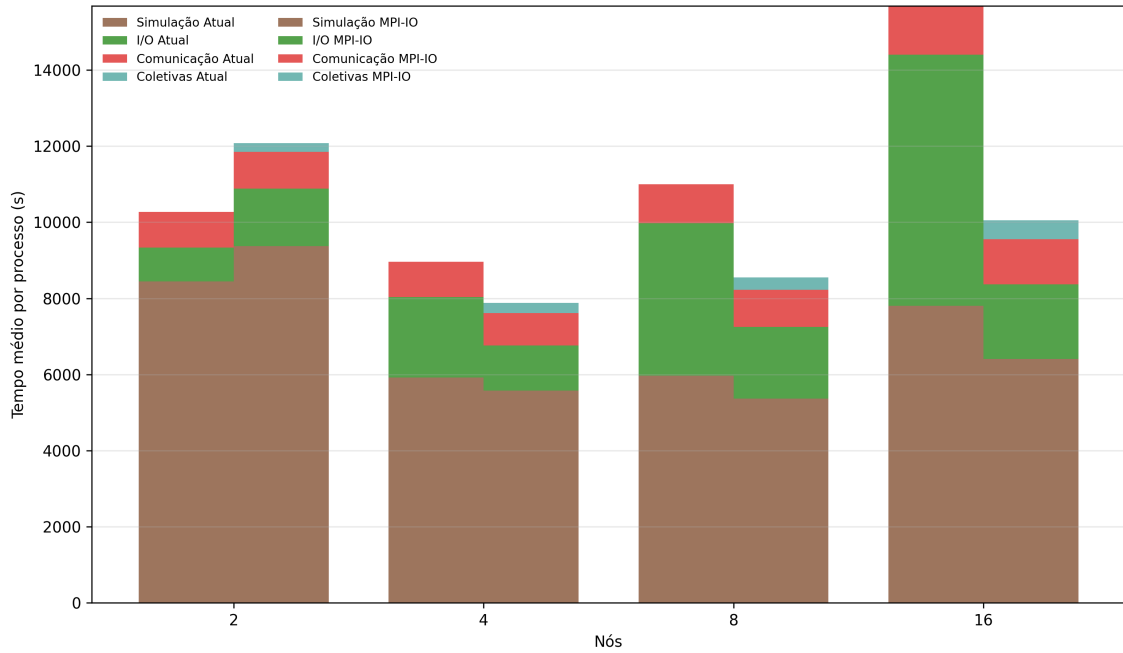
Figura 4.3: Decomposição do tempo médio por processo das implementações atual e MPI-IO no Experimento SDumont.
