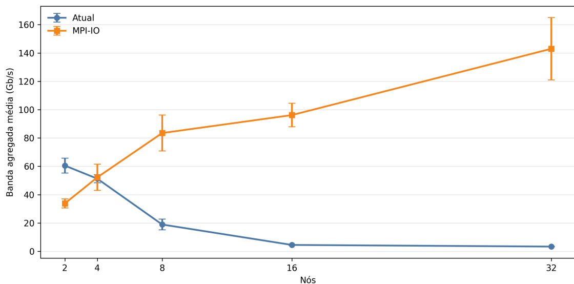
Figura 4.5: Banda agregada média no Experimento AWS.
