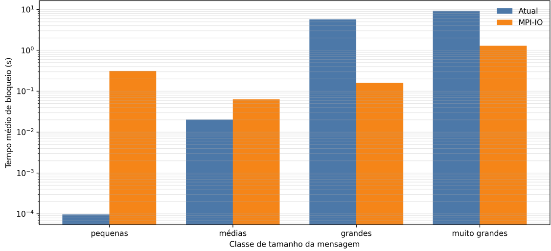
Figura 4.4: Tempo médio de bloqueio das operações de envio por tamanho de mensagem nas implementações atual e MPI-IO no Experimento SDumont (escala logarítmica).
