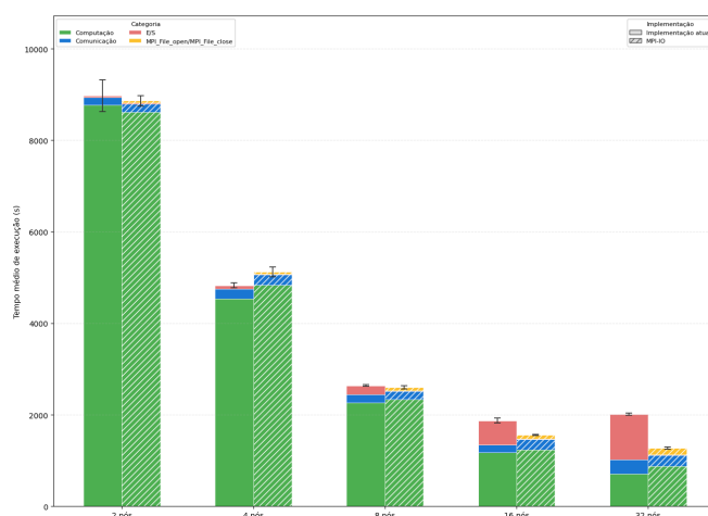
Figura 5. Tempo de execução no Experimento AWS.
