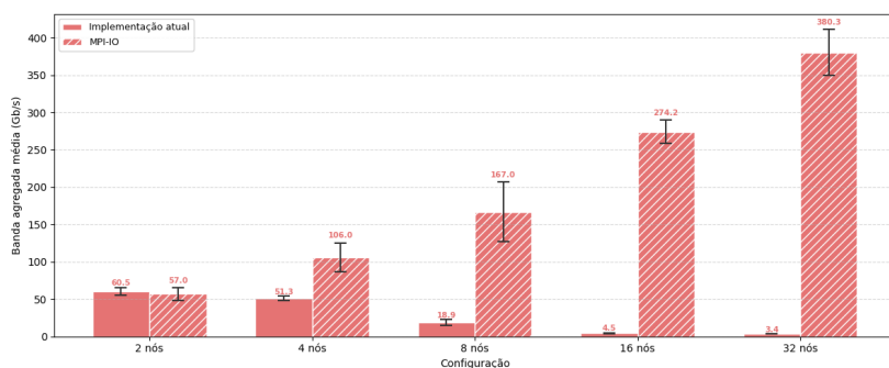
Figura 4. Banda agregada percebida no Experimento AWS.
