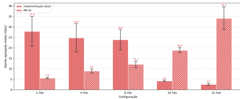
Figura 7. Banda agregada percebida no Experimento SDumont.
