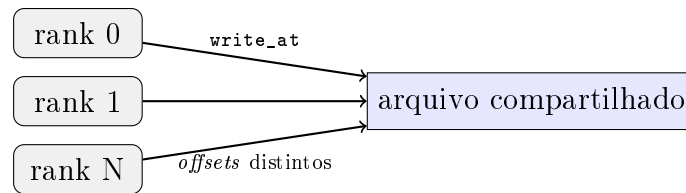
Figura 2.2: Relação entre comunicação ponto a ponto e E/S paralela. No modelo centralizado, os resultados passam por um processo escritor; no modelo MPI-IO, os próprios processos escrevem diretamente no arquivo.
