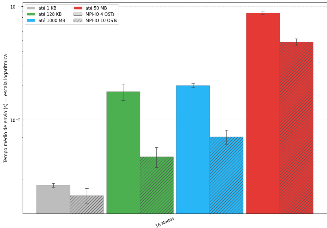
Figura 4.8: Experimento com diferentes nós OSTs.
