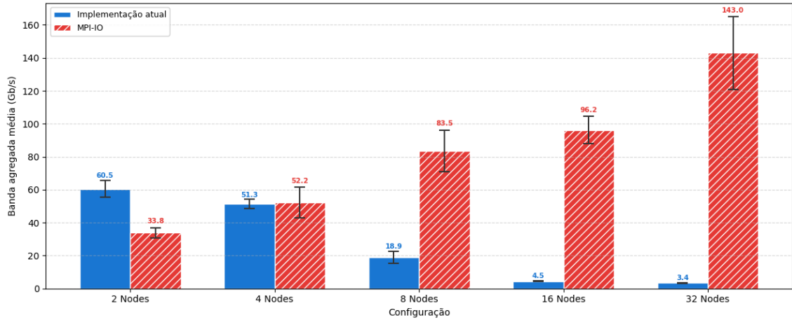
Figura 4.5: Banda agregada média no Experimento AWS.
