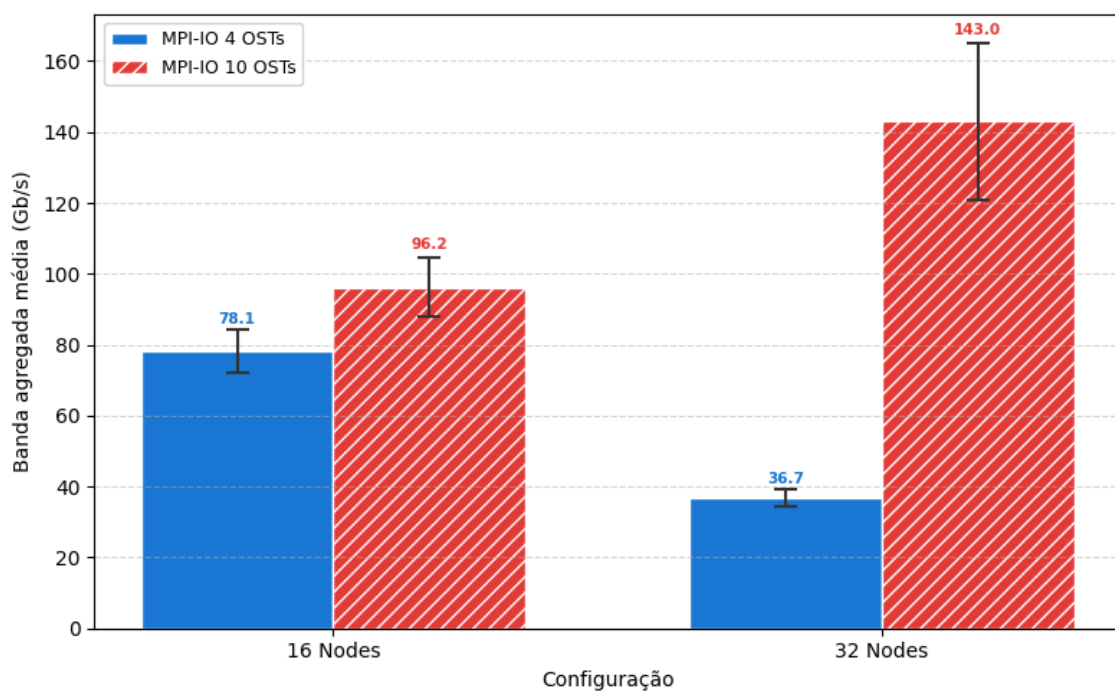
Figura 4.9: Banda agregada média para configurações MPI-IO com 4 e 10 OSTs.
