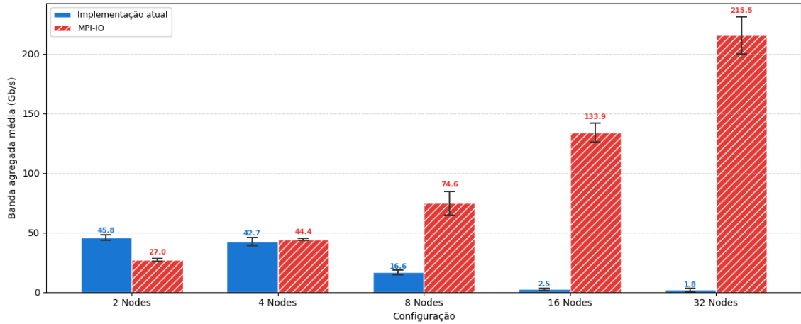
Figura 4.2: Banda agregada média no Experimento AWS.
