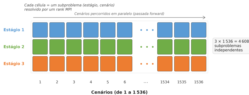
Figura 2.1: Estrutura de cenários e estágios do SDDP nos experimentos desta dissertação. Cada célula corresponde a um subproblema (estágio, cenário). Os cenários são mutuamente independentes e podem ser distribuídos entre ranks MPI, caracterizando uma aplicação bag-of-tasks .
