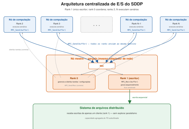
Figura 1. Arquitetura atual de E/S do SDDP: o rank 0 distribui tarefas e o rank 1 concentra todas as operações de escrita.
