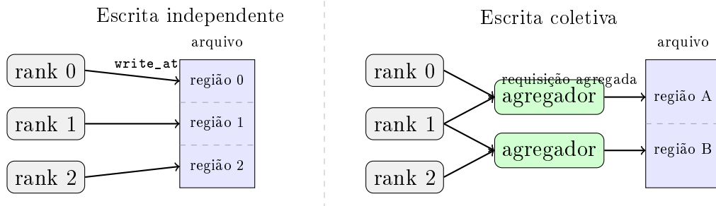
Figura 2.2: Diferença entre escritas independentes e coletivas em MPI-IO. Escritas independentes preservam autonomia dos ranks ; escritas coletivas permitem agregação e reordenação das requisições pela biblioteca MPI-IO.
