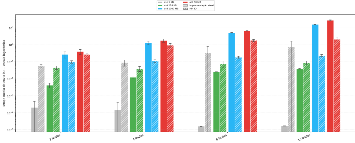
Figura 4.4: Tempo médio de bloqueio das operações de envio por tamanho de mensagem nas implementações atual e MPI-IO no Experimento SDumont (escala logarítmica).
