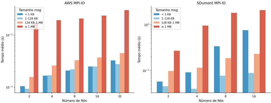
Tempo Médio de I/O por Faixa de Tamanho (MPI-IO)
