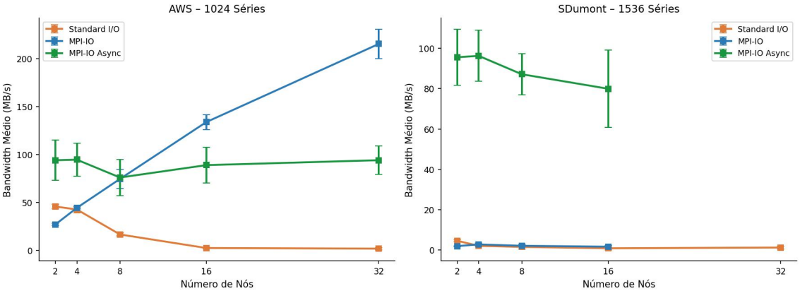
Largura de Banda de I/O vs. Nós (maior = melhor)
