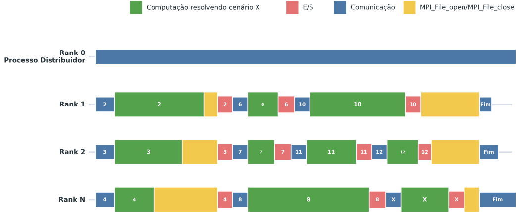
Figura 3. Linha de tempo da simulação final do SDDP com MPI-IO: os ranks trabalhadores executam cenários, sincronizam na abertura coletiva, realizam escritas independentes e sincronizam no fechamento.
