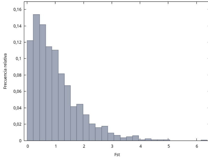
Figura 1: Los 2000 valores del F bajo H_0 cierta con n = 506 . La masa está entre 0 y 2; la cola derecha llega más allá de 5. El valor crítico F_c(3, 502) = 2,62 deja a su derecha el 5,5 % de las réplicas.
