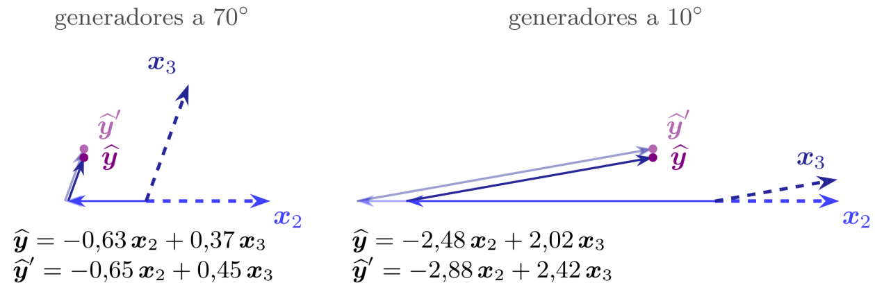
Figura 2: Dos regresores en desviaciones y de longitud 1 (a trazos), que forman 70^\circ a la izquierda y 10^\circ a la derecha, y el mismo punto \hat{\mathbf{y}} en los dos paneles. Los tramos continuos son su descomposición \hat{\beta}_2 \mathbf{x}_2 + \hat{\beta}_3 \mathbf{x}_3 : primero \hat{\beta}_2 \mathbf{x}_2 , horizontal y hacia la izquierda porque \hat{\beta}_2 < 0 , y después \hat{\beta}_3 \mathbf{x}_3 hasta \hat{\mathbf{y}} . \hat{\mathbf{y}}' es el ajuste que daría otra muestra: dista 0,07 de \hat{\mathbf{y}} en la dirección perpendicular a \mathbf{x}_2 , y su descomposición va en color más claro. A 70^\circ las coordenadas cambian poco, lo mismo que el ajuste; a 10^\circ cambian 0,40 cada una y en sentidos opuestos, casi seis veces el desplazamiento del ajuste: el factor es 1/\sin 10^\circ .
