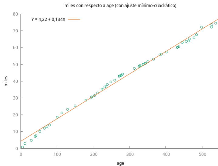
Figura 1: miles frente a age : los cincuenta y siete coches están casi sobre una recta. La correlación es 0,9965.
