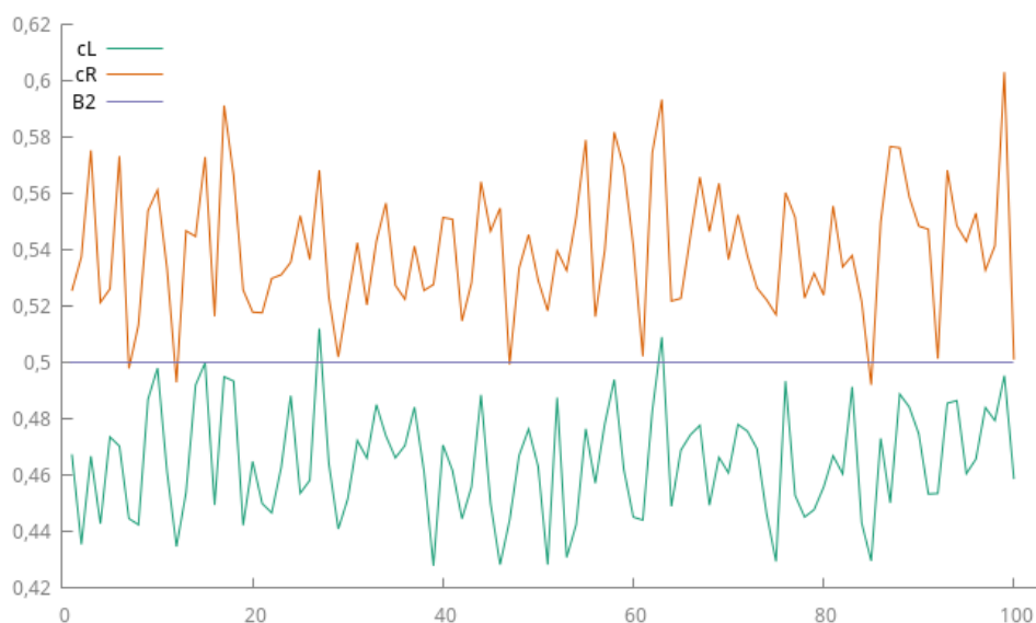
Figura 1: Los cien primeros intervalos de confianza al 95%: extremo inferior y superior de cada uno, frente al verdadero \beta_2 = 0,5 (línea horizontal). Los intervalos que no lo contienen son aquellos en los que una de las dos líneas cruza la horizontal.
