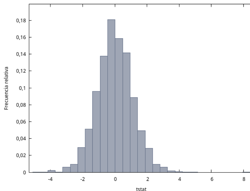
Figura 2: Histograma de los 4000 estadísticos t = (\hat{\beta}_2 - 0,5)/ee(\hat{\beta}_2) , calculados bajo la hipótesis cierta. Sus cuantiles del 2,5% y del 97,5% caen donde los sitúa la t_{10} , no donde los sitúa la normal.
