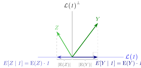
Figura 1: Proyección de la variable aleatoria Y sobre el subespacio generado por la variable constante 1 . El escalar de la proyección es E(Y) (la esperanza matemática o valor esperado), y el vector proyectado es la v.a. constante E[Y|1] = E(Y)1 (la esperanza condicional).
