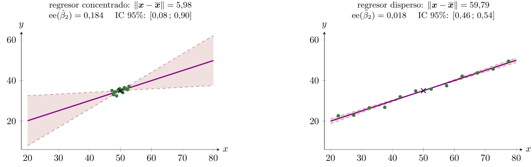
Figura 4: Dos ajustes con la misma muestra de perturbaciones, el mismo n = 12 y el mismo residuo, y por tanto el mismo \mathfrak{s} = 1,10 . Lo único distinto es cuánto se separan los valores del regresor. La zona sombreada es el haz de rectas cuyas pendientes caen en el intervalo de confianza al 95 %, dibujadas pivotando sobre el centroide, por donde la recta de regresión pasa siempre. Diez veces más largo el regresor en desviaciones, diez veces más estrecho el haz.
