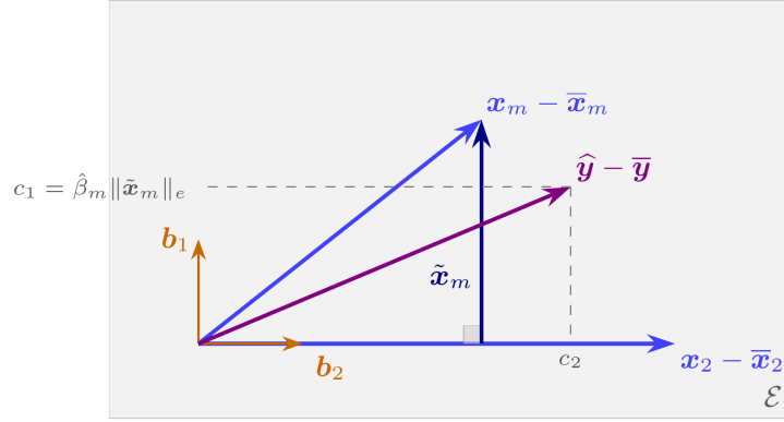
Figura 5: El plano \mathcal{E} visto de frente, con k = 3 : dos regresores en desviaciones, no ortogonales entre sí. La parte propia \tilde{x}_m es la componente de x_m - \bar{x}_m ortogonal al otro regresor; está dibujada desplazada, como residuo, desde la proyección hasta la punta, pero como vector parte del origen, en la dirección de b_1 , que es su dirección normalizada; b_2 es la dirección del otro regresor. La coordenada del ajuste en desviaciones sobre b_1 es c_1 = \hat{\beta}_m \|\tilde{x}_m\|_e , de donde (9).
