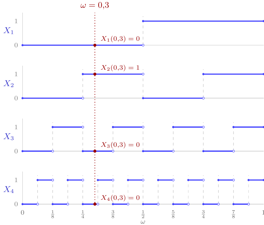
Figura 2: Las cuatro primeras monedas como funciones sobre \Omega = [0, 1] (la figura del apéndice de la lección 11, con una moneda más). Cada una vale 0 en los intervalos impares de longitud 2^{-n} y 1 en los pares. La línea de puntos es el suceso elemental \omega = 0,3 , que en base dos empieza 0,0100...: cruz, cara, cruz, cruz. Un \omega es una tirada infinita. Es la única figura del documento que dibuja dónde vale qué una variable aleatoria, y muestra por qué no se insiste en ello: cada fila es más apretada que la anterior, y pocas más abajo la función ya no se lee. Por eso las demás figuras dibujan las variables aleatorias como vectores.
