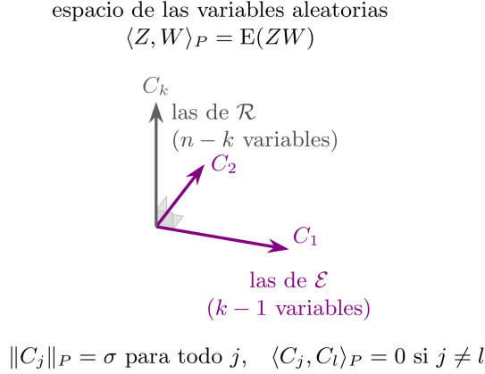
Figura 8: El Resultado 1 en el otro espacio. Las C_j son elementos del espacio de las variables aleatorias, con el producto escalar \langle Z, W \rangle_P = E(ZW) de la lección 9: una familia ortogonal cuyos n - 1 miembros miden lo mismo, \sigma . Las k - 1 de \mathcal{E} y las n - k de \mathcal{R} se distinguen solo por el vector de la base al que corresponden. Aquí no hay datos ni vectores de \mathbb{R}^n : la figura es un esquema de tres de las n - 1 variables.
