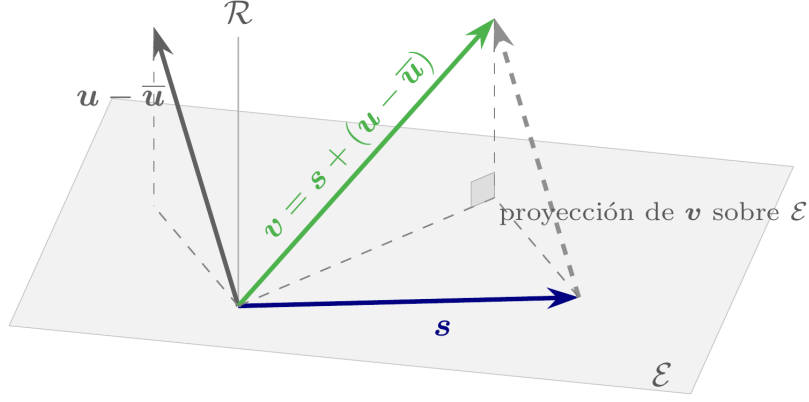
Figura 7: Una realización \omega , dibujada en \mathbb{R}^n . Los tres vectores parten del origen: \mathbf{s} es la realización de (S_1, \dots, S_n) y está en \mathcal{E} ; \mathbf{u} - \bar{\mathbf{u}} es la realización de las perturbaciones centradas, con componente en \mathcal{E} (su proyección, en línea de puntos) y en \mathcal{R} ; \mathbf{v} es su suma, y la copia a guiones de \mathbf{u} - \bar{\mathbf{u}} trasladada a la punta de \mathbf{s} solo muestra la regla del paralelogramo. La proyección de \mathbf{v} sobre \mathcal{E} es \mathbf{s} más la proyección del ruido; su componente en \mathcal{R} es solo la del ruido, porque \mathbf{s} no tiene. Por eso las coordenadas de \mathbf{v} sobre los vectores de la base de \mathcal{R} son c_j y sobre los de \mathcal{E} son d_j + c_j , donde d_j y c_j son los valores en \omega de D_j y C_j . Bajo H_0 : \beta_2 = \dots = \beta_k = 0 , \mathbf{s} = \mathbf{0} y \mathbf{v} es el ruido centrado.
