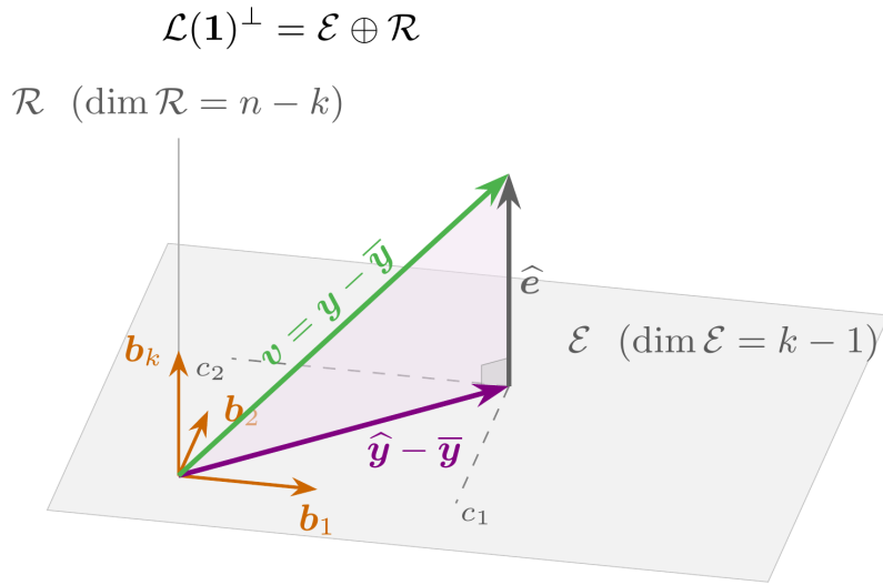
Figura 4: Los dos subespacios de \mathcal{L}(\mathbf{1})^\perp , la base adaptada y el primer triángulo. El plano representa \mathcal{E} (de dimensión k-1 ) y la vertical \mathcal{R} (de dimensión n-k ); \mathbf{b}_1, \mathbf{b}_2 son vectores de la base en \mathcal{E} y \mathbf{b}_k en \mathcal{R} . El vector de datos en desviaciones \mathbf{v} , de longitud \|\mathbf{v}\|_e = \sqrt{\sum_{\mathcal{E}} c_j^2 + \sum_{\mathcal{R}} c_j^2} , se descompone en su proyección sobre \mathcal{E} , el ajuste en desviaciones, de longitud \|\hat{\mathbf{y}} - \bar{\mathbf{y}}\|_e = \sqrt{\sum_{\mathcal{E}} c_j^2} , y su componente en \mathcal{R} , el residuo, de longitud \|\hat{\mathbf{e}}\|_e = \sqrt{\sum_{\mathcal{R}} c_j^2} . Todo son vectores de datos: ninguna variable aleatoria.
