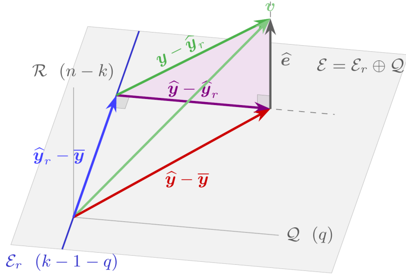
Figura 6: El tercer triángulo. Los tres ejes parten del origen: dentro de \mathcal{E} , la recta azul es \mathcal{E}_r y la perpendicular a ella dentro del plano es \mathcal{Q} ; la vertical es \mathcal{R} . El ajuste restringido en desviaciones es la proyección de \mathbf{v} sobre \mathcal{E}_r . El triángulo está dibujado desplazado, con el vértice en la punta de \hat{\mathbf{y}}_r - \bar{\mathbf{y}} : sus lados son vectores que en realidad parten del origen, y las líneas a guiones son los ejes \mathcal{Q} y \mathcal{R} trasladados en paralelo hasta él. Lo que el modelo completo añade, \hat{\mathbf{y}} - \hat{\mathbf{y}}_r , vive en \mathcal{Q} y tiene longitud \|\hat{\mathbf{y}} - \hat{\mathbf{y}}_r\|_e = \sqrt{\sum_{\mathcal{Q}} c_j^2} = \sqrt{\text{SRC}_r - \text{SRC}} ; el residuo vive en \mathcal{R} y tiene longitud \|\hat{\mathbf{e}}\|_e = \sqrt{\sum_{\mathcal{R}} c_j^2} = \sqrt{\text{SRC}} ; la hipotenusa es el residuo restringido, de longitud \|\mathbf{y} - \hat{\mathbf{y}}_r\|_e = \sqrt{\text{SRC}_r} . Es la figura del Pitágoras anidado de la lección 13 con los subespacios nombrados.
