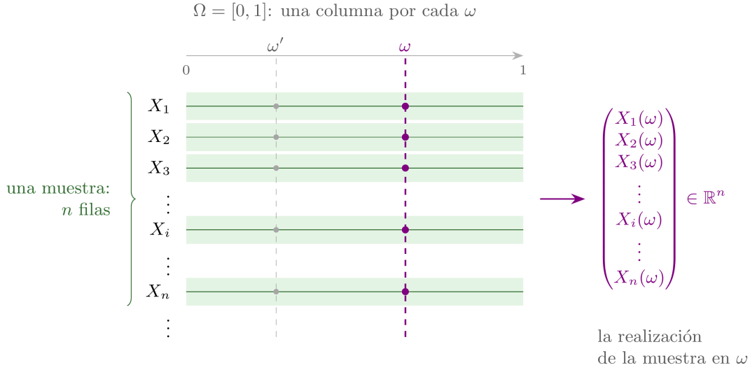
Figura 3: La matriz de copias. Cada fila es una copia de la variable, una función sobre \Omega ; la matriz continúa hacia abajo indefinidamente. Elegir n filas es tomar una muestra; elegir una columna es fijar un \omega ; las dos cosas a la vez dan el vector (X_1(\omega), \dots, X_n(\omega)) de \mathbb{R}^n . Los datos observados son una columna; una simulación Monte Carlo recorre otras columnas, \omega', \omega'', \dots , con las mismas filas.
