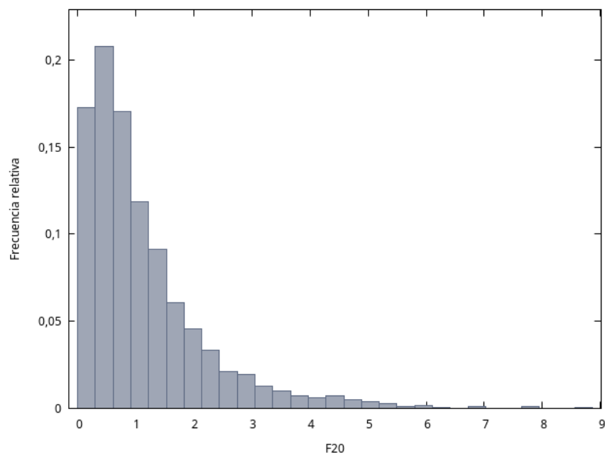
Figura 2: Los 2000 valores del F bajo H_0 cierta con n = 20 . La cola derecha es más pesada que con n = 506 : llega casi hasta 9, y el valor crítico al 5 % es 3,24 en lugar de 2,62 (el cuantil empírico del 95 % está en 3,28).
