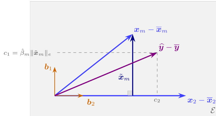
Figura 5: El plano \mathcal{E} visto de frente, con k = 3 : dos regresores en desviaciones, no ortogonales entre sí. La parte propia \tilde{\mathbf{x}}_m es la componente de \mathbf{x}_m - \bar{\mathbf{x}}_m ortogonal al otro regresor; está dibujada desplazada, como residuo, desde la proyección hasta la punta, pero como vector parte del origen, en la dirección de \mathbf{b}_1 , que es su dirección normalizada; \mathbf{b}_2 es la dirección del otro regresor. La coordenada del ajuste en desviaciones sobre \mathbf{b}_1 es c_1 = \hat{\beta}_m \|\tilde{\mathbf{x}}_m\|_e , de donde (9).
