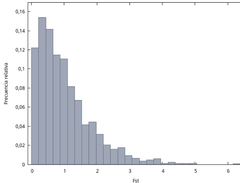
Figura 1: Los 2000 valores del F bajo H_0 cierta con n = 506 . La masa está entre 0 y 2; la cola derecha llega más allá de 5. El valor crítico F_c(3, 502) = 2,62 deja a su derecha el 5,5 % de las réplicas.
