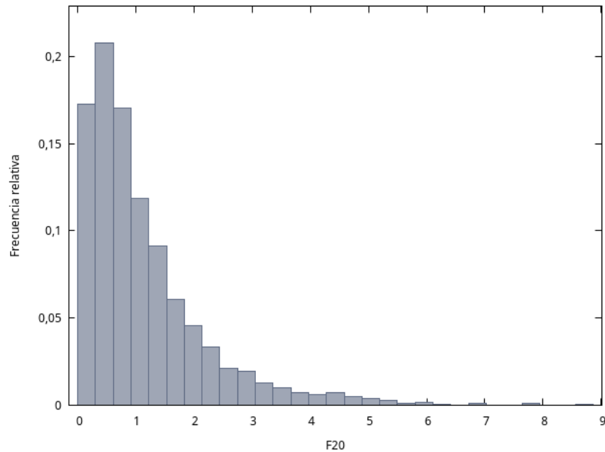
Figura 2: Los 2000 valores del F bajo H_0 cierta con n = 20 . La cola derecha es más pesada que con n = 506 : llega hasta 9, y el 5 % superior empieza en 3,24 en lugar de 2,62.
