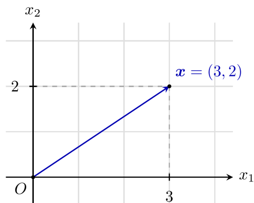
Figura 1: Ejemplo. El vector \mathbf{x} = (3, 2) \in \mathbb{R}^2 es la lista (3, 2) , que corresponde al punto del plano con primera coordenada 3 y segunda coordenada 2.
