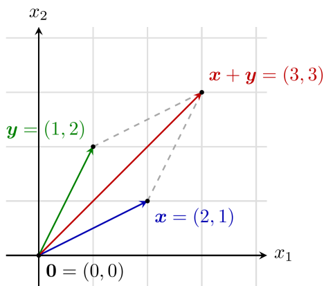
Figura 2: Ejemplo con \mathbf{x} = (2, 1) , \mathbf{y} = (1, 2) , \mathbf{x} + \mathbf{y} = (3, 3) .
