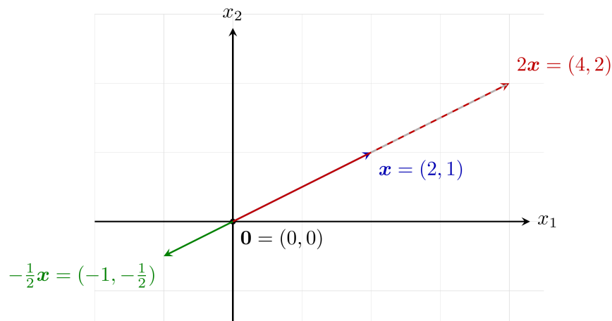
Figura 3: Ejemplo con \mathbf{x} = (2, 1) , 2\mathbf{x} = (4, 2) , -\frac{1}{2}\mathbf{x} = (-1, -\frac{1}{2}) .
