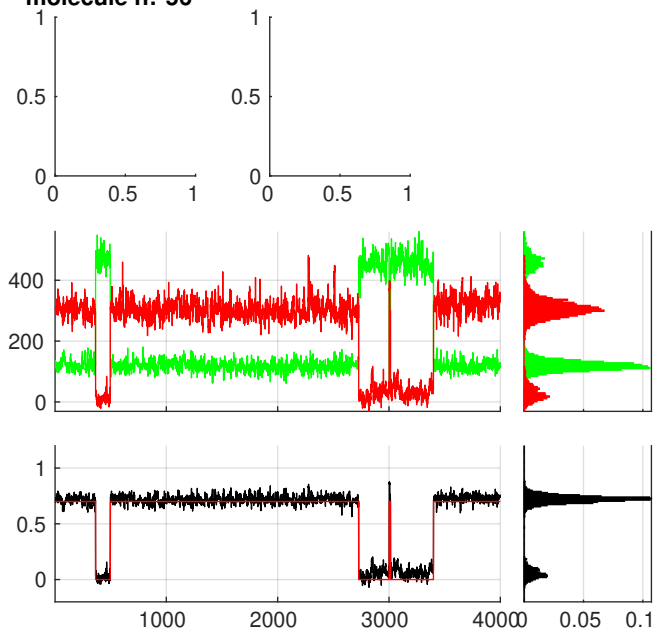
molecule n:°58
