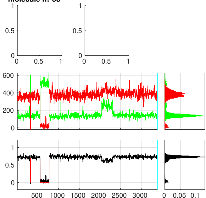
molecule n:°60
