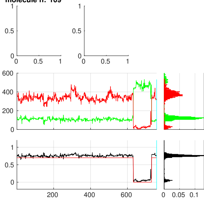
molecule n:°111
