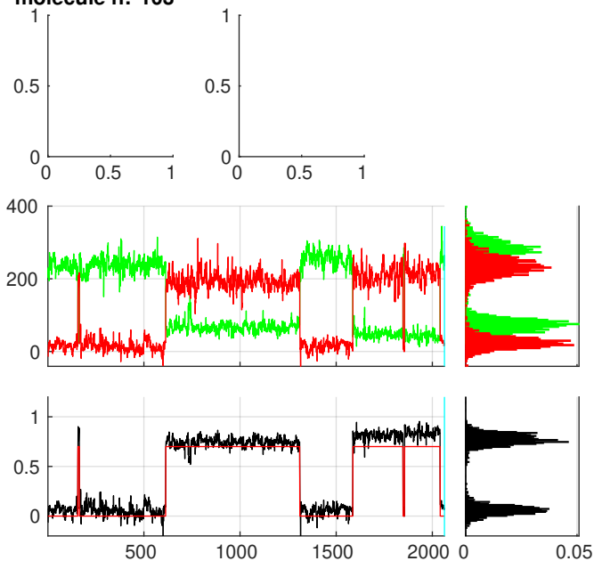
molecule n:°105
