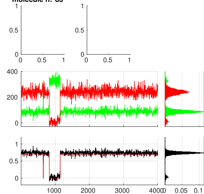
molecule n:°83
