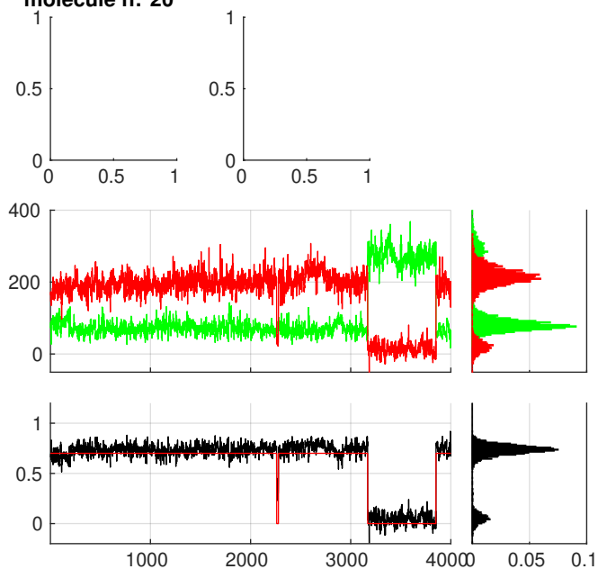
molecule n:°22
