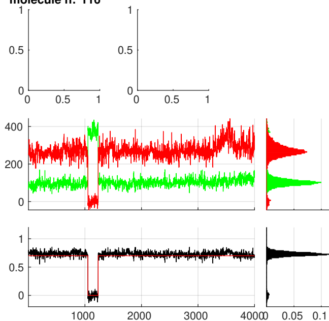
molecule n:°118
