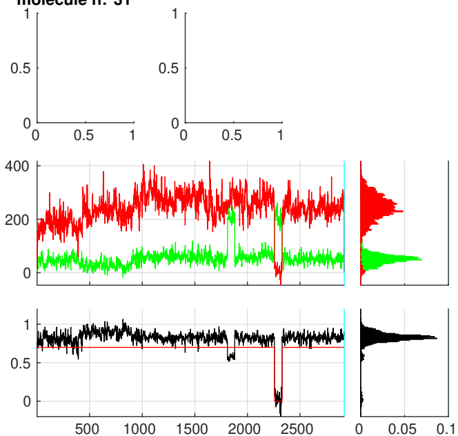
molecule n:°33
