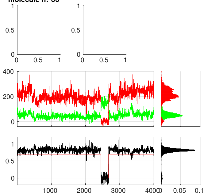
molecule n:°36
