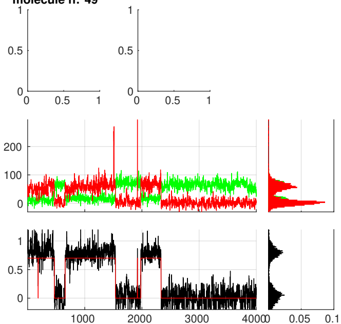
molecule n:°51
