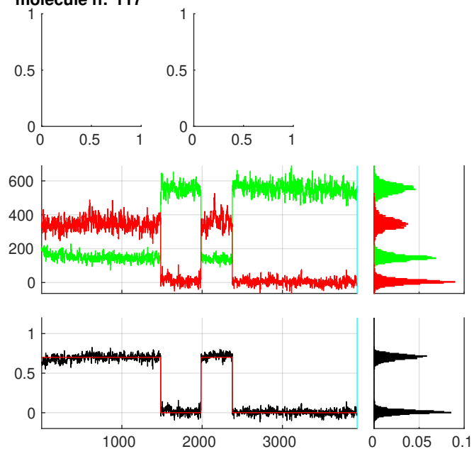
molecule n:°117
