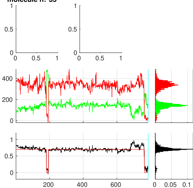
molecule n:°35
