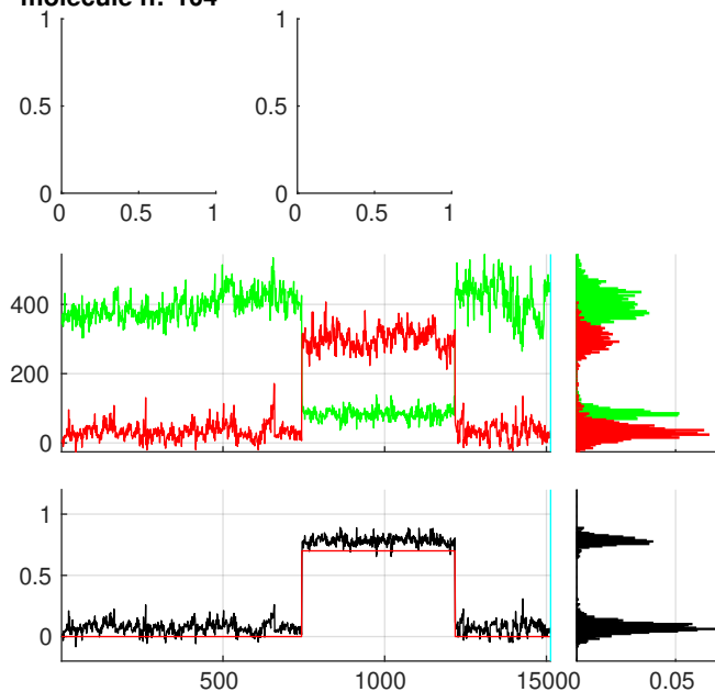
molecule n:°106
