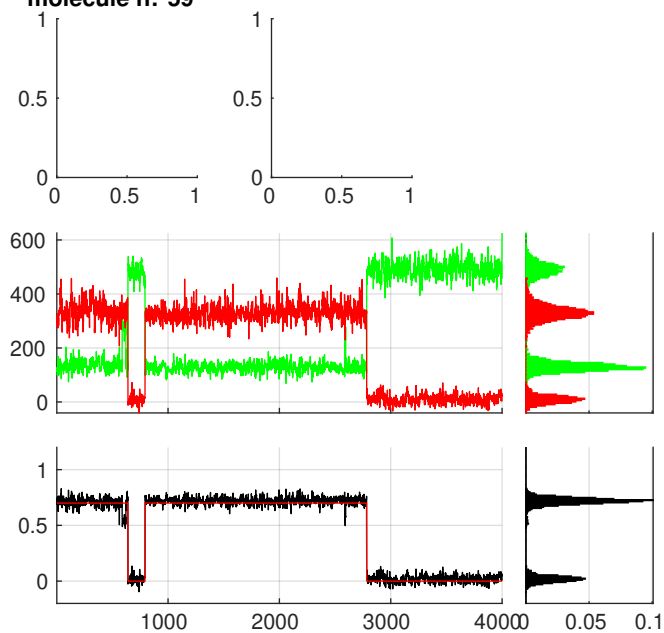
molecule n:°59
