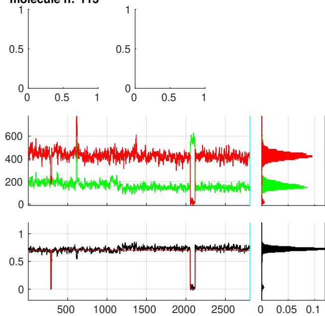
molecule n:°113
