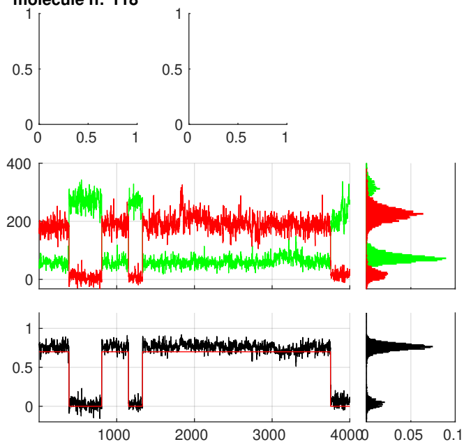
molecule n:°118
