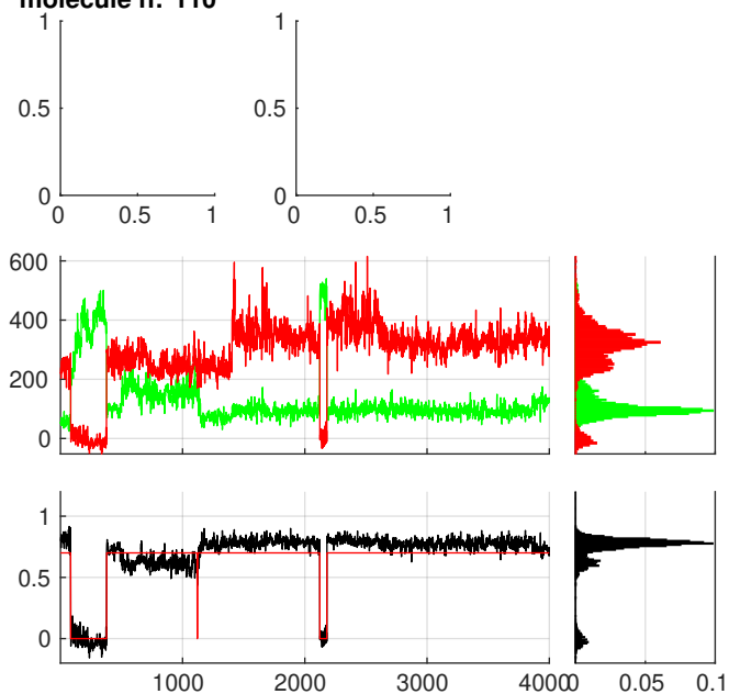
molecule n:°112
