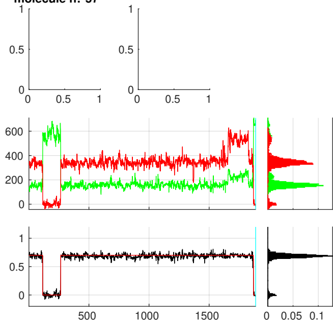
molecule n:°59
