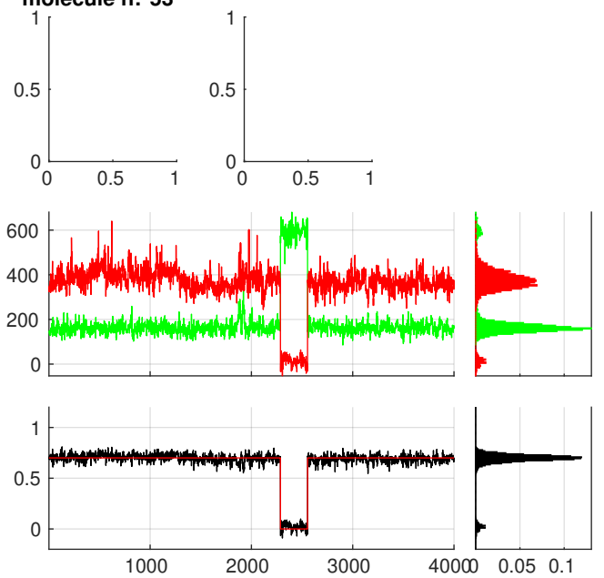
molecule n:°53
