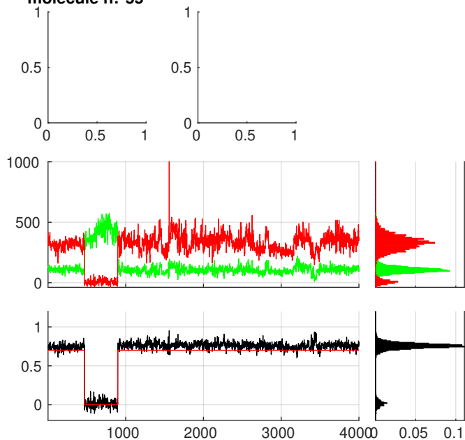
molecule n:°57
