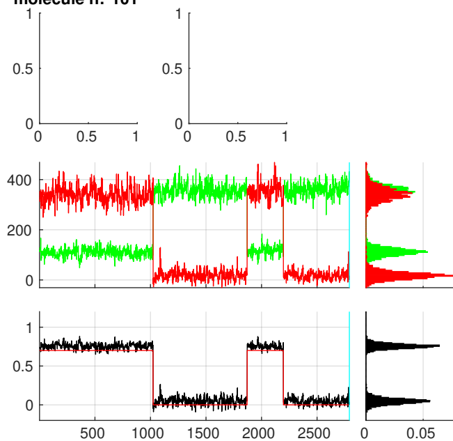
molecule n:°101
