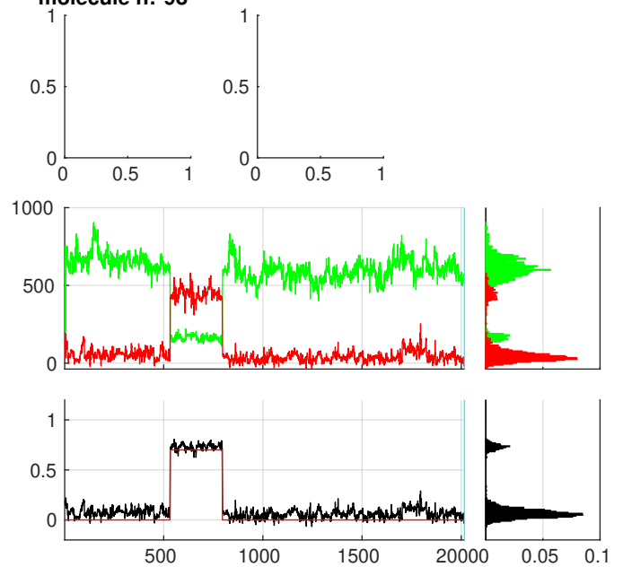
molecule n:°100
