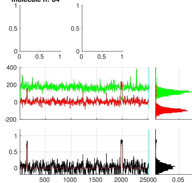
molecule n:°84
