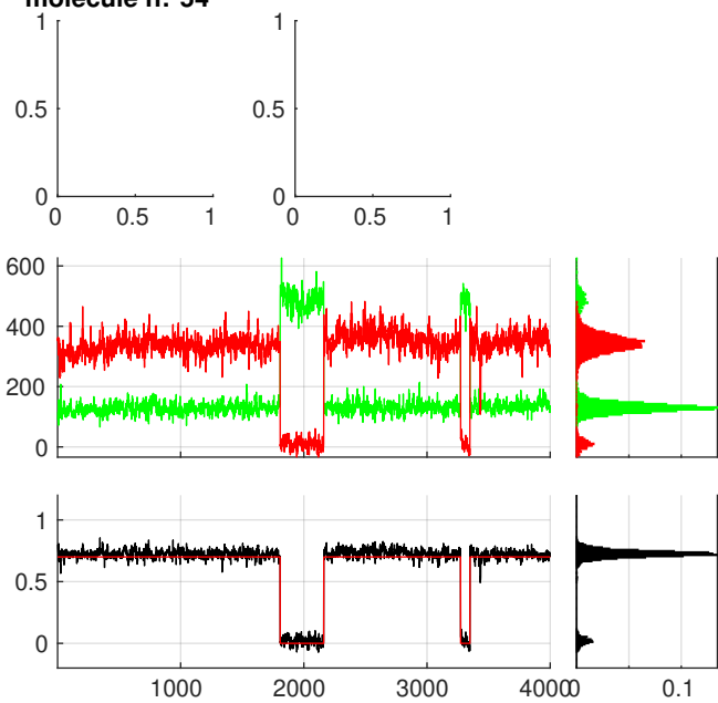
molecule n:°54
