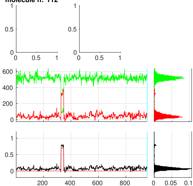
molecule n:°114
