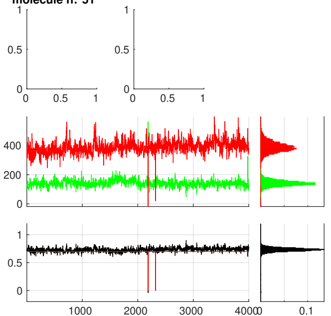
molecule n:°53
