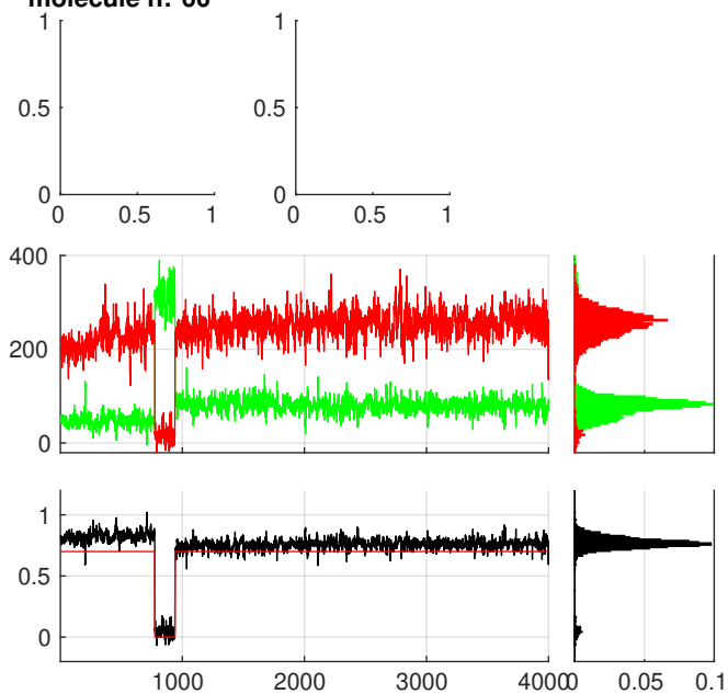
molecule n:°60
