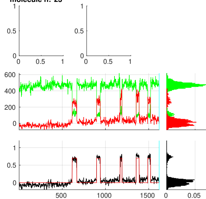
molecule n:°23
