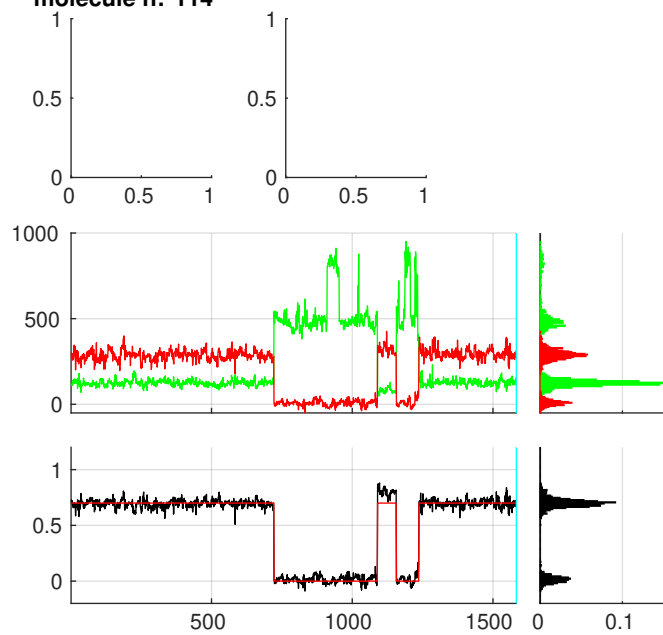
molecule n:°114
