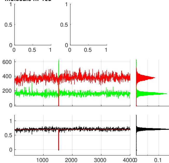
molecule n:°108
