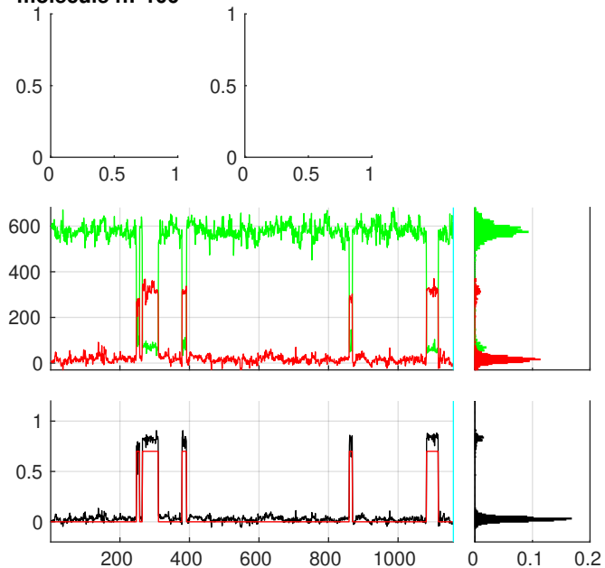
molecule n:°108
