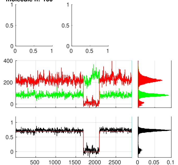
molecule n:°102
