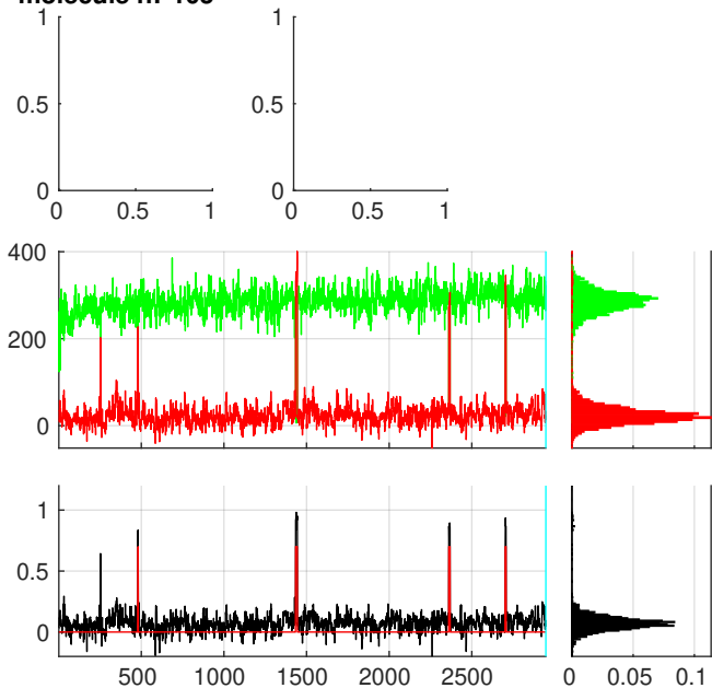
molecule n:°107
