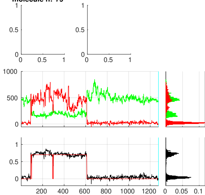
molecule n:°81
