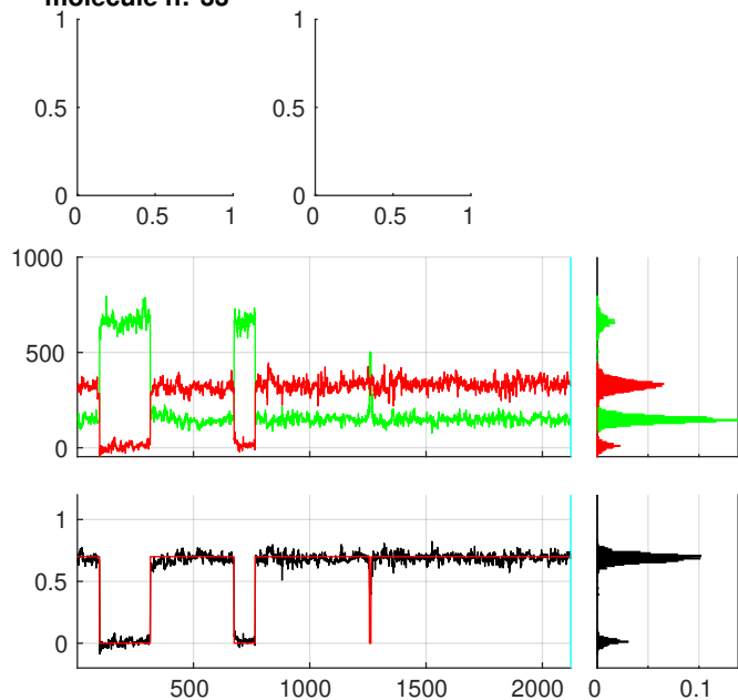
molecule n:°35
