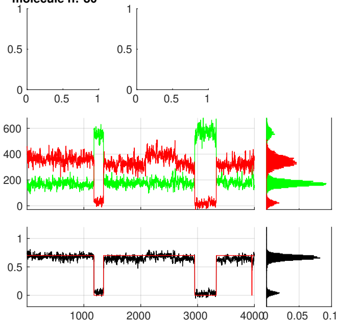
molecule n:°82
