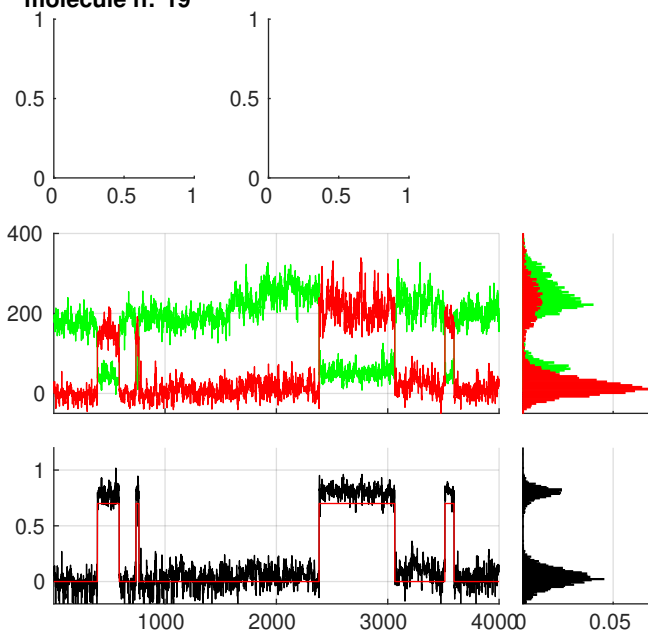
molecule n:°21
