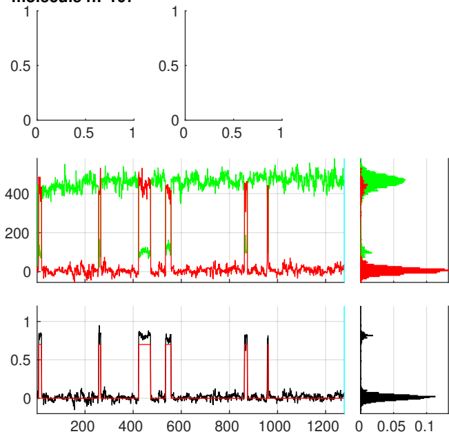
molecule n:°107
