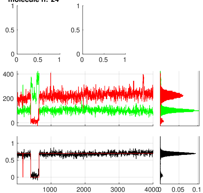
molecule n:°24
