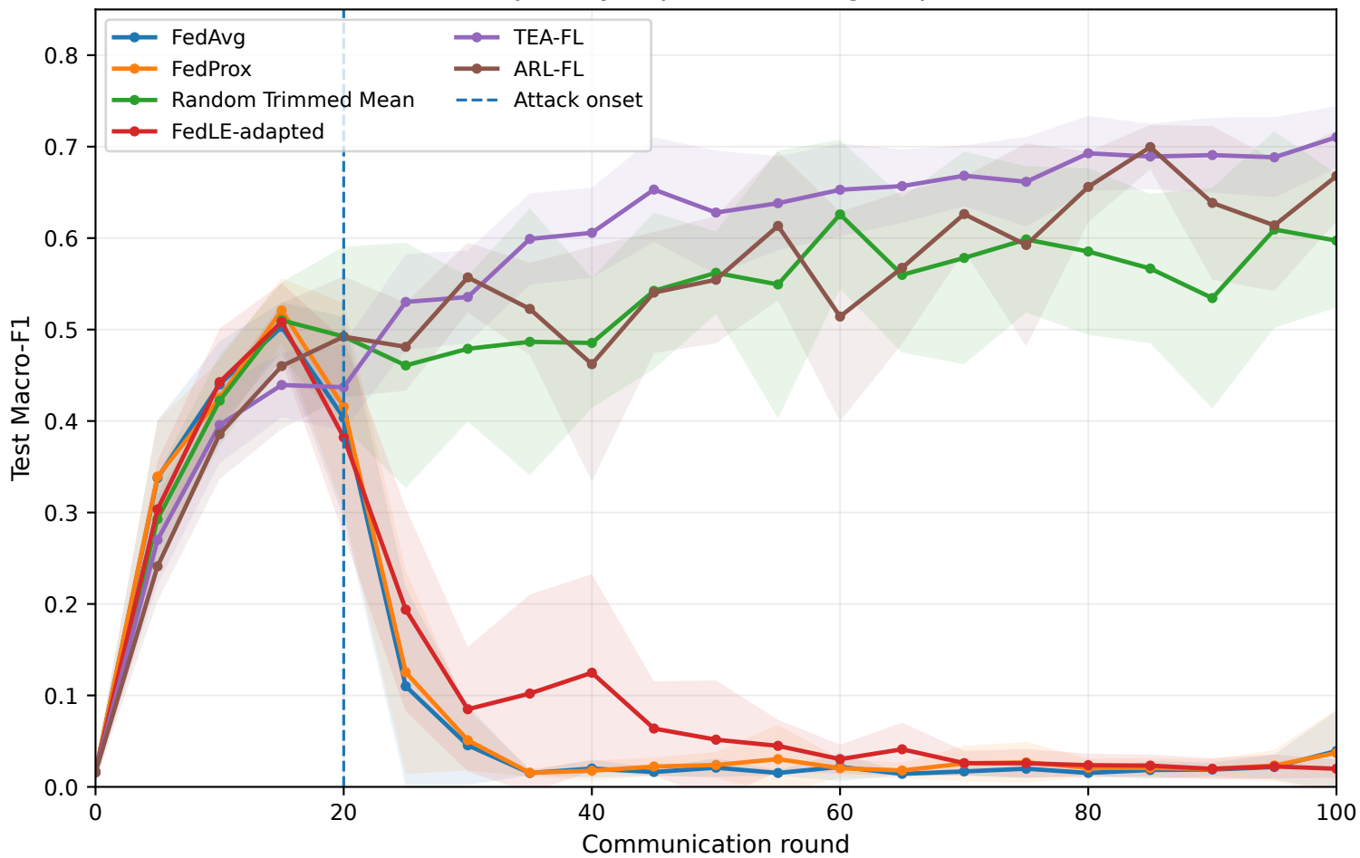
PAMAP2 trajectory: \alpha = 1.0 , sign-flip \mu = 0.2
