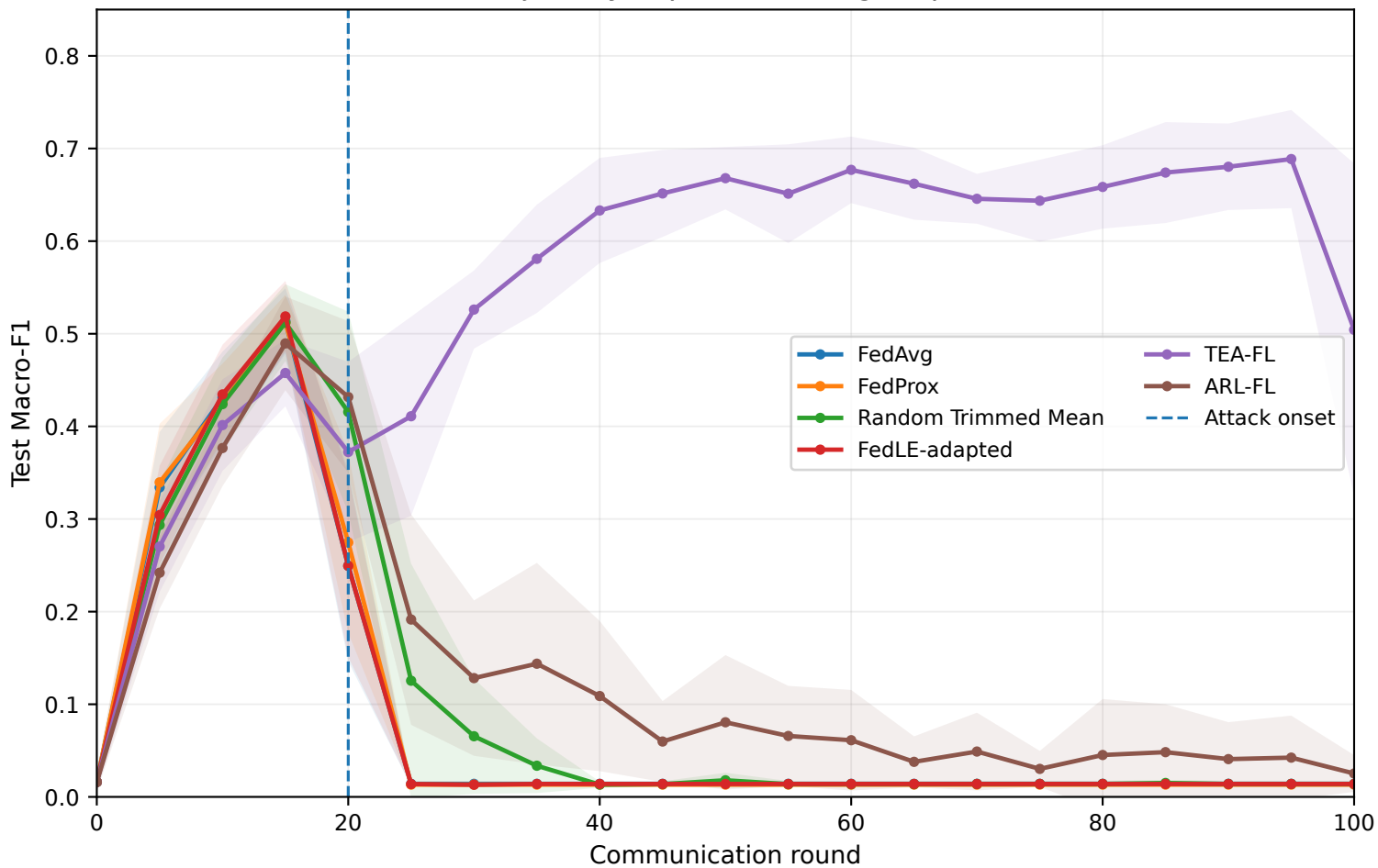
PAMAP2 trajectory: \alpha = 1.0 , sign-flip \mu = 0.4
