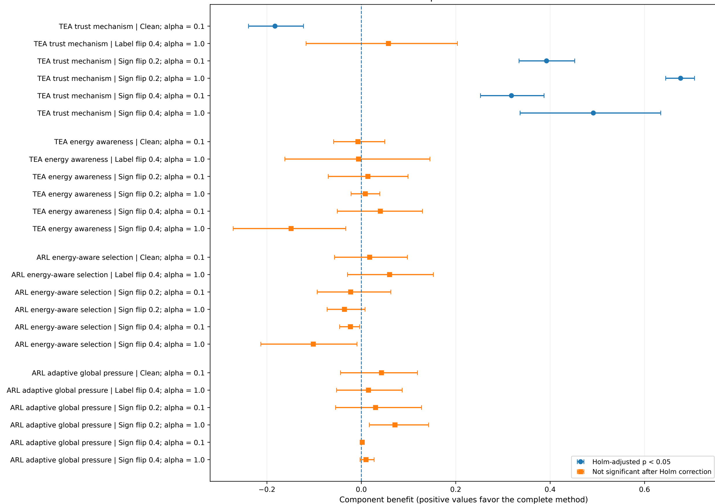
PAMAP2 component effects on Macro-F1
