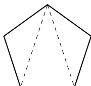
pentágono: 3 triángulos
