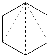
hexágono: 4 triángulos
