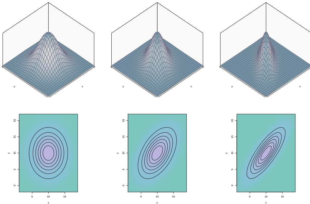
Abbildung 4.16: Dichte von gemeinsamer Normalverteilung
