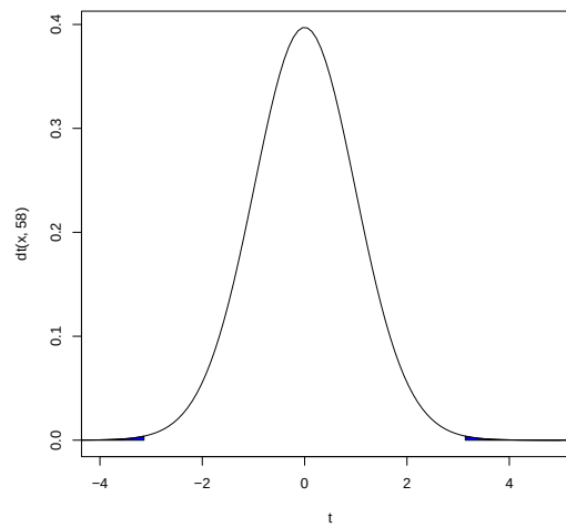
Abbildung 8.2: t -Verteilung mit df = 58 mit p -Wert bei beobachteter Statistik t = 3.14
