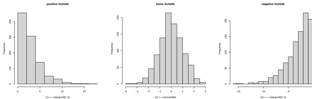
Abbildung 5.9: Verteilungen mit positiver, keiner und negativer Schiefe
