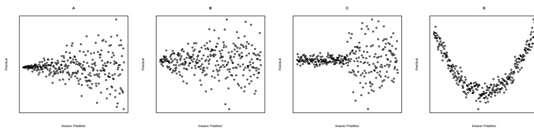
Abbildung 13.6: A: linear wachsende Standardabweichung, B: nicht-linear wachsende Standardabweichung, C: zwei Gruppen mit unterschiedlicher Varianz, D: fehlender quadratischer Term im Modell.
