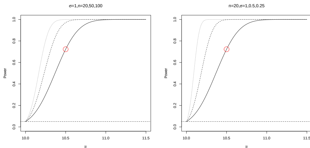
Abbildung 8.4: Power-Funktion eines einseitigen z -Tests, mit H_0 : \mu \leq 10 . Links: n = 20 (—), 50 (--), 100 (...) und \sigma = 1 . Rechts: n = 20 und \sigma = 1 (—), 0.5 (--), 0.25 (...).
