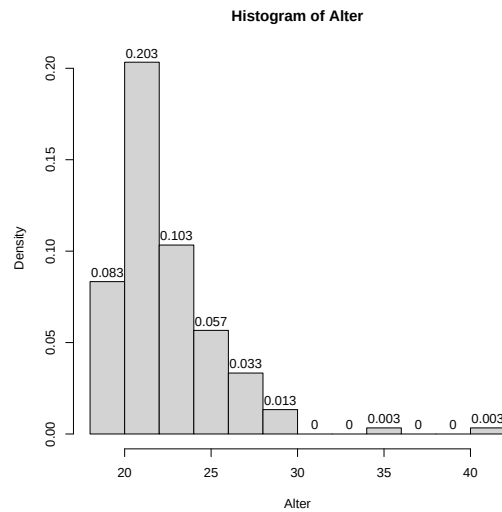
Abbildung 5.2: Relative Häufigkeitsverteilung (links geschlossene Klassen, Klassenbreite 2)
