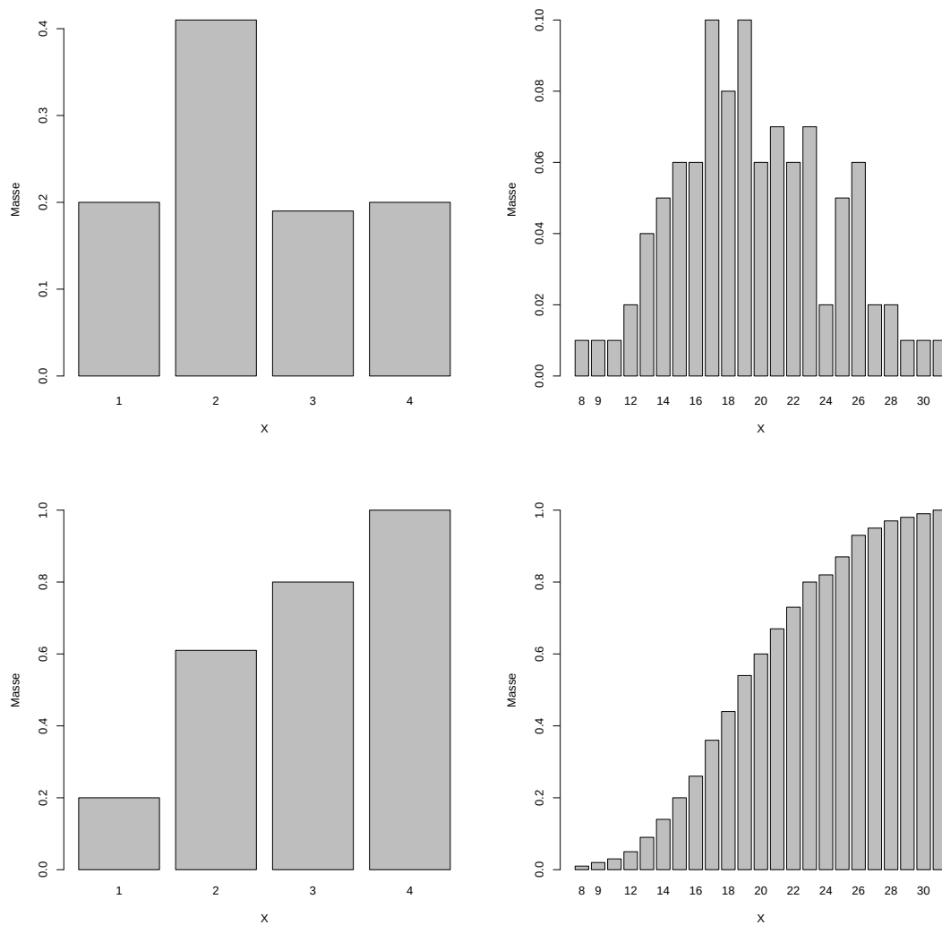
Abbildung 4.2: Diskrete Zufallsvariable. Gewichtsfunction (oben) und kumulative Verteilungsfunktion (unten)
