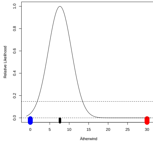
Abbildung 8.8: Relative Likelihood, gegeben die Daten. Schwarz: Der beobachtete Wert ist = 7.62 und hat maximale relative Likelihood. Der Schwellenwert von 0.145 für die relative Likelihood entspricht einem approximativen 95%-CI von (1.77, 13.46) . Die obere Grenze des CI ist klar weiter weg von \delta = 30 als die untere Grenze von \delta = 0 .
