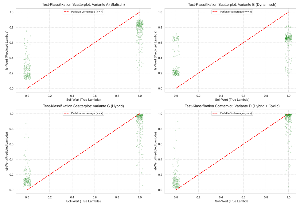
Vergleich der MixUp-Regressoren: Ist- vs. Soll-Werte auf dem Test-Split (Reine Sätze)
