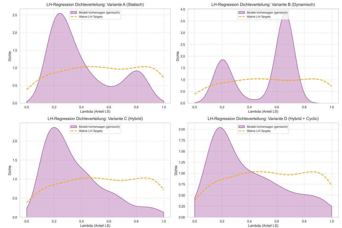
Vergleich der MixUp-Regressoren: Vorhersage- vs. Target-Verteilung auf dem gemischten Lebenshilfe-Set
