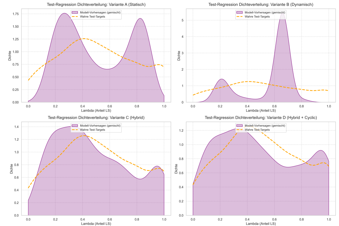
Vergleich der MixUp-Regressoren: Vorhersage- vs. Target-Verteilung auf dem gemischten Test-Split
