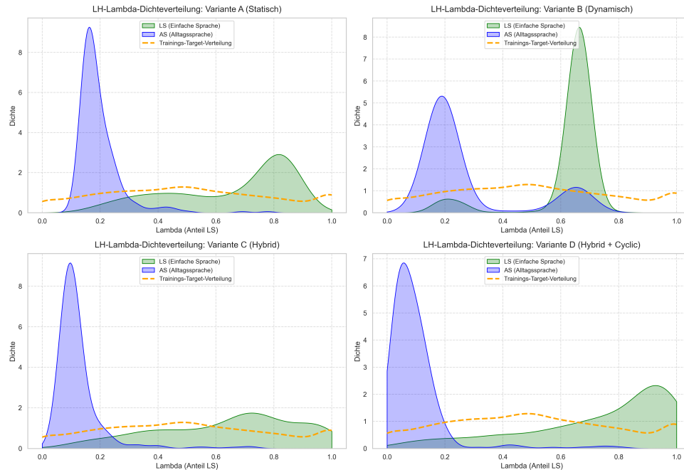
Vergleich der MixUp-Regressoren auf dem Lebenshilfe-Datensatz (Reine Sätze) vs. Trainings-Target-Verteilung
