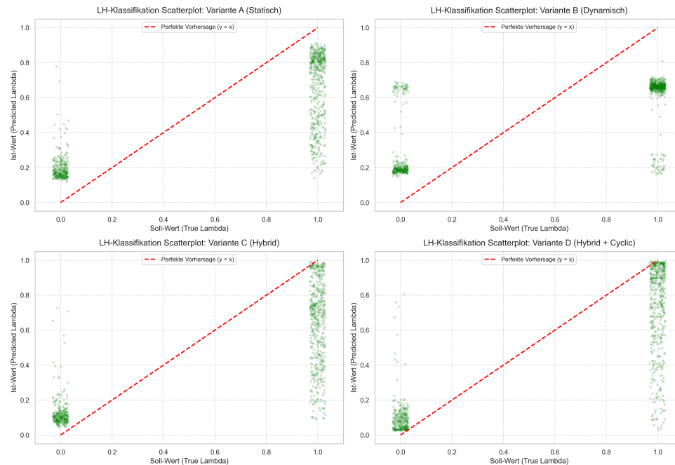
Vergleich der MixUp-Regressoren: Ist- vs. Soll-Werte auf dem Lebenshilfe-Set (Reine Sätze)
