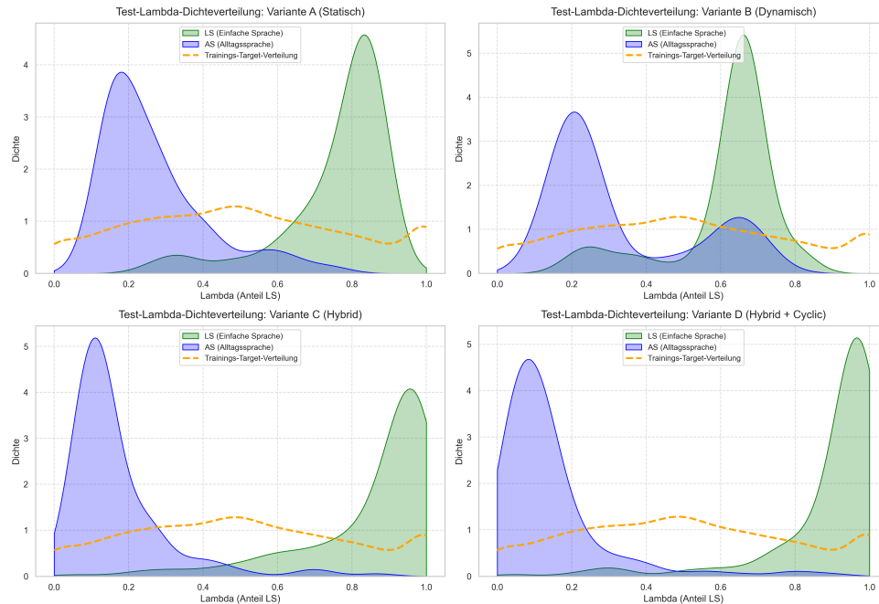
Vergleich der MixUp-Regressoren auf dem Test-Split (Reine Sätze) vs. Trainings-Target-Verteilung
