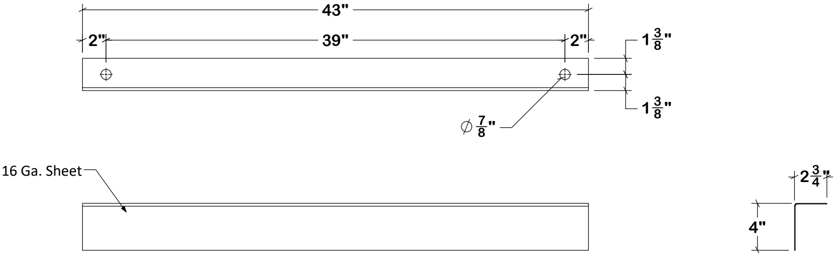
Small Riser Pan - QTY (2)
