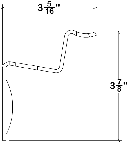
Typ Wallgrab Bracket - QTY (8)
