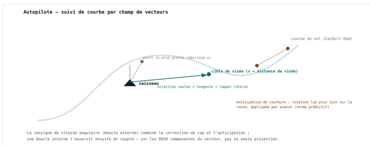
Figure 7 — suivi de courbe par champ de vecteurs, avec anticipation de courbure
