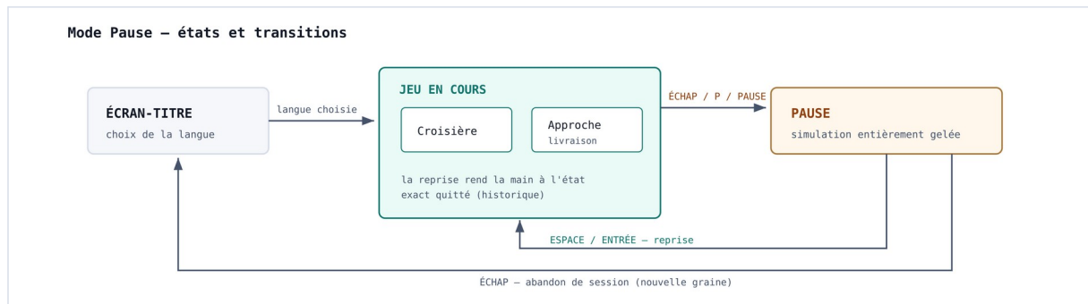
Figure 17 — états et transitions du mode Pause
