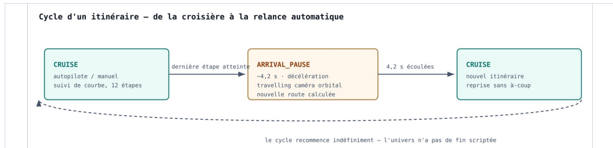
Figure 11 — cycle croisière / pause d'arrivée / nouvelle croisière
