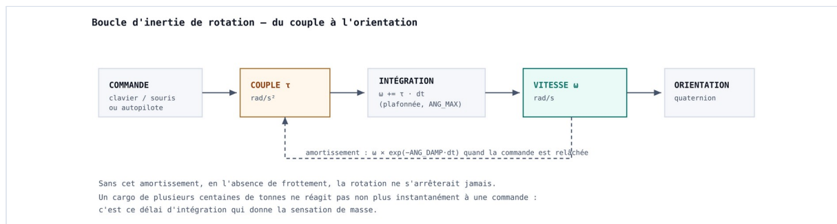
Figure 6 — boucle d'inertie de rotation
