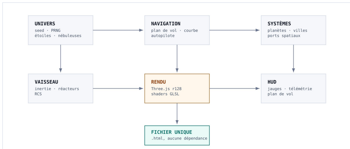
Figure 1 — vue d'ensemble des grands modules du simulateur
