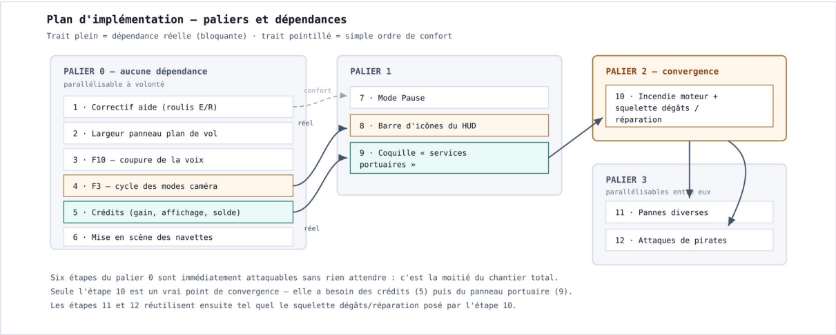
Figure 19 — paliers d'implémentation et dépendances
