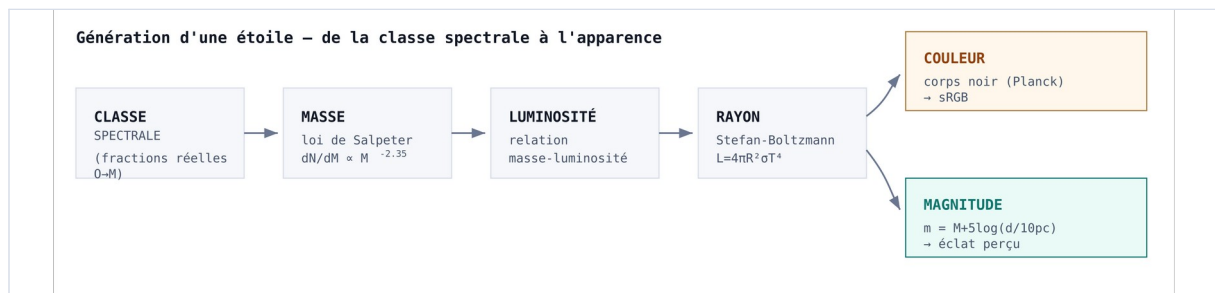
Figure 2 — pipeline de génération d'une étoile
