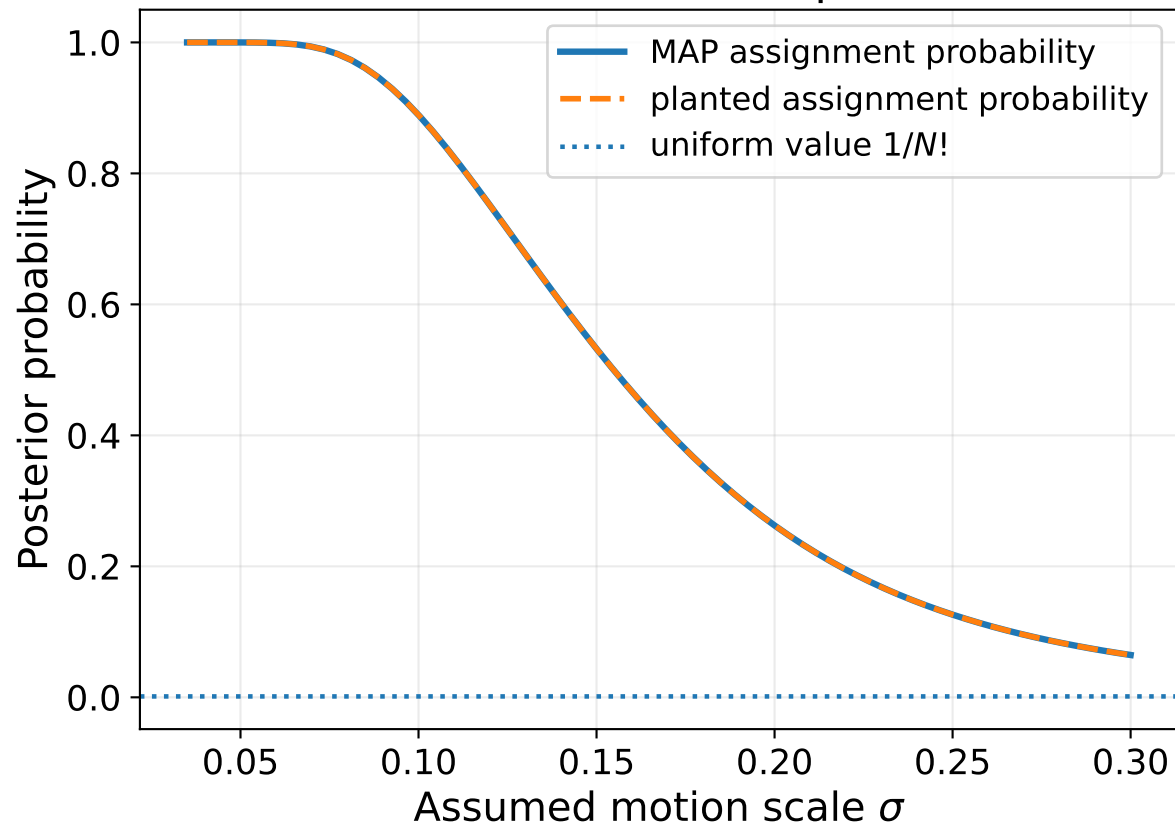
Stable MAP, uncertain posterior
