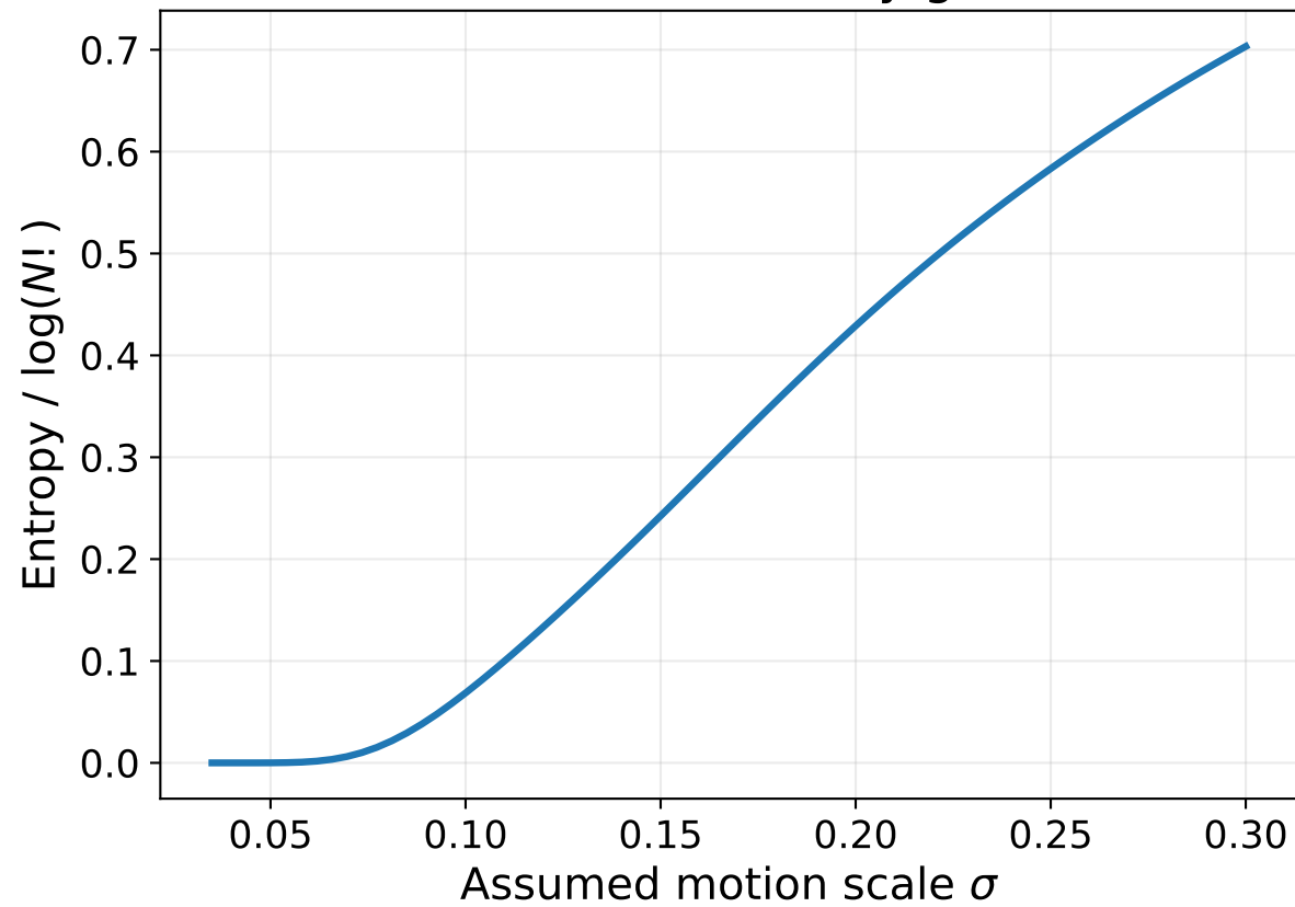
Posterior uncertainty grows
