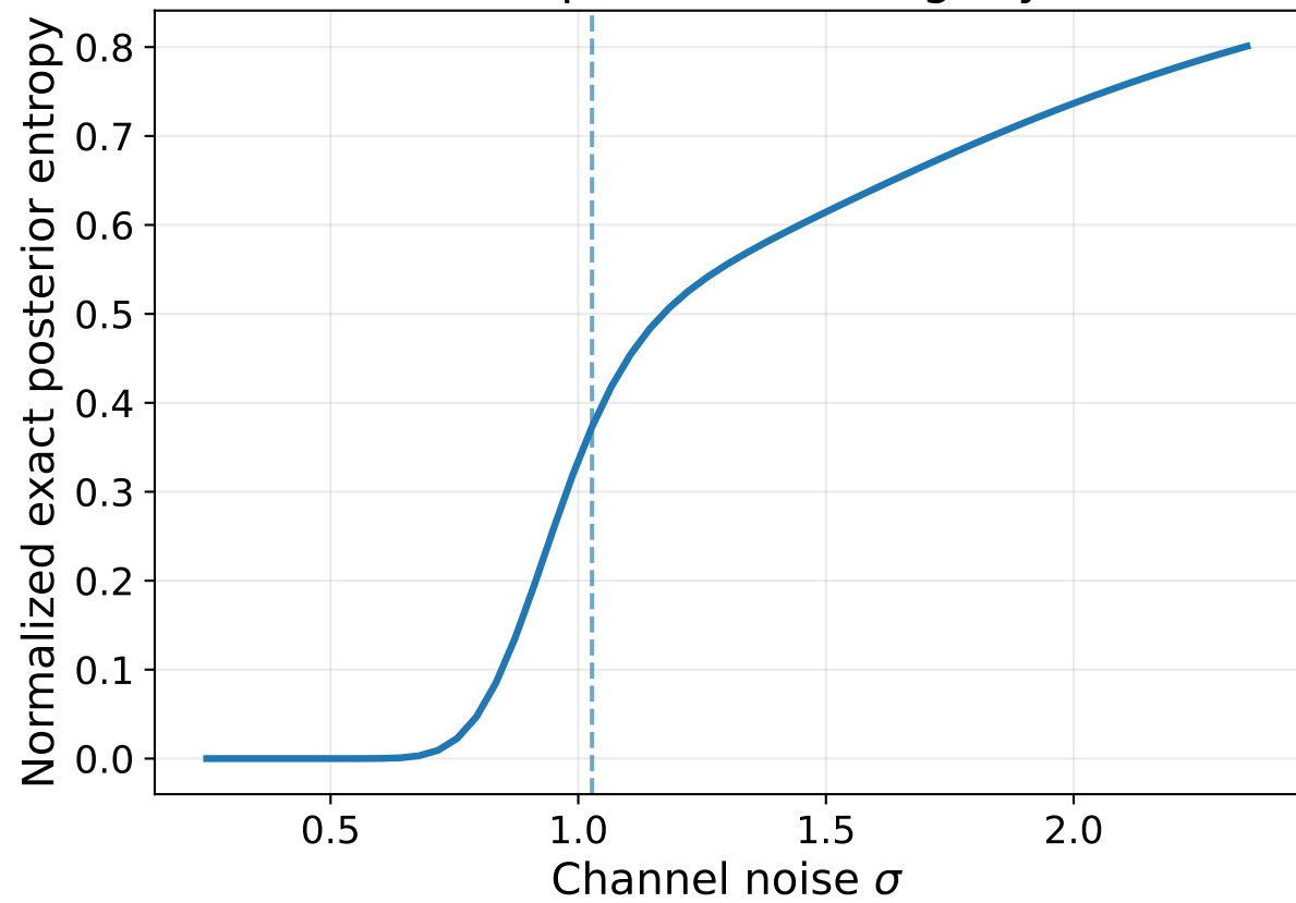
Exact posterior ambiguity
