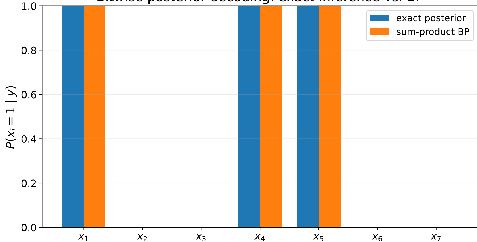
Bitwise posterior decoding: exact inference vs. BP
