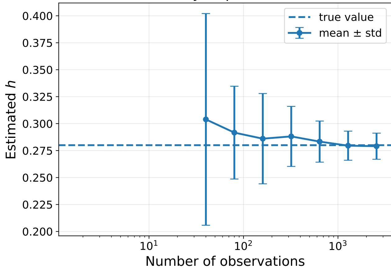
Recovery of parameter h
