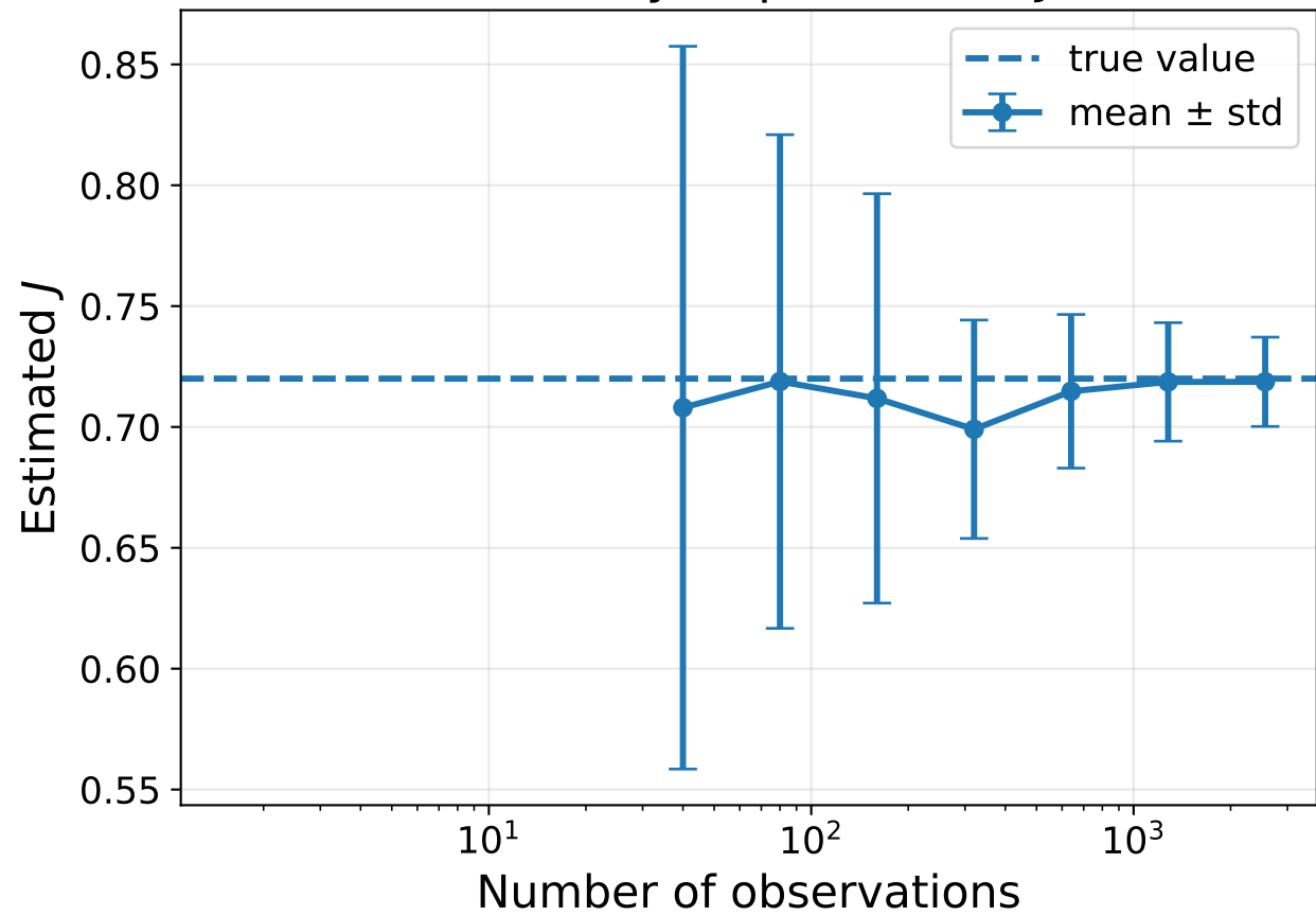
Recovery of parameter J
