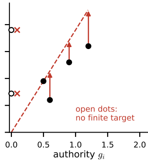
(d) BOTC: add noise upper bound
