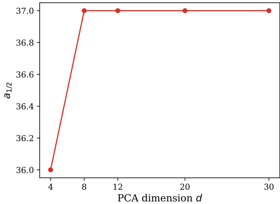
(b) Half-life vs PCA dimension
