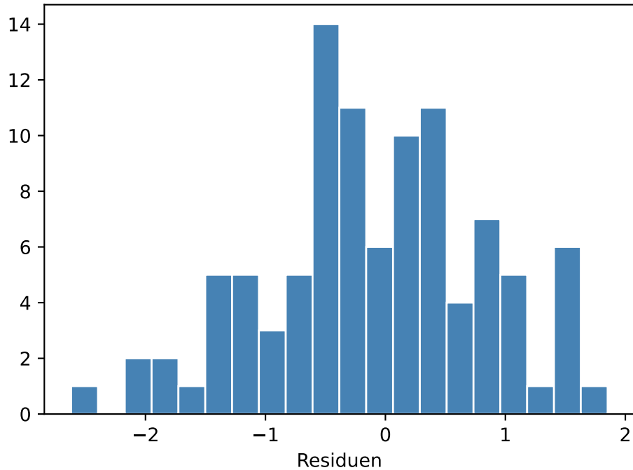
Histogramm der Residuen
