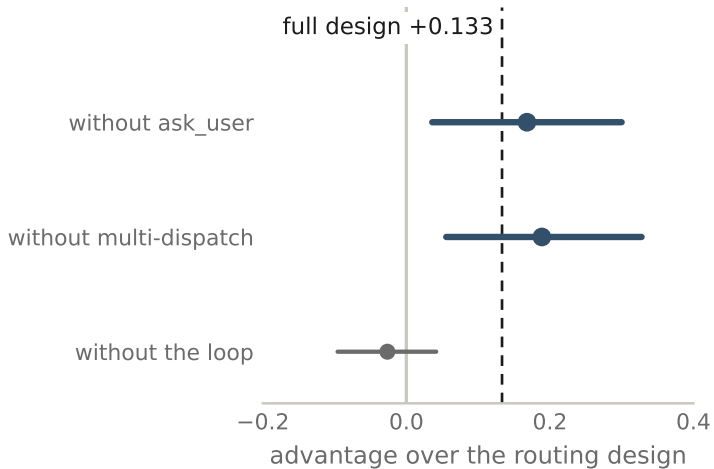
on-device (llama3.1:8b)
