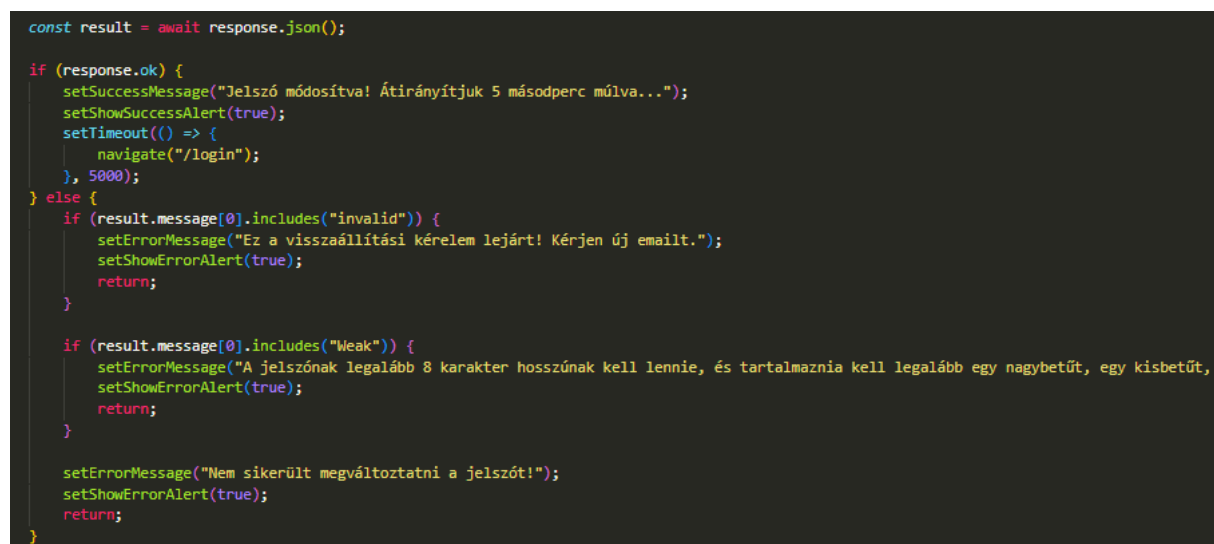
22. ábra: Üzenetek
