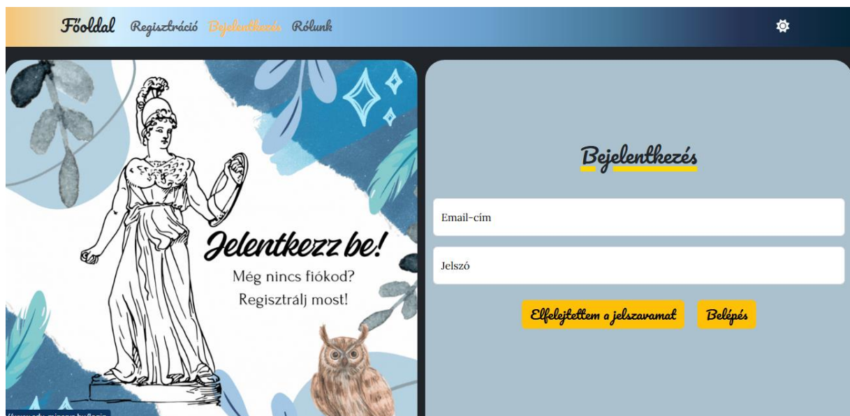
8. ábra: Bejelentkezés
