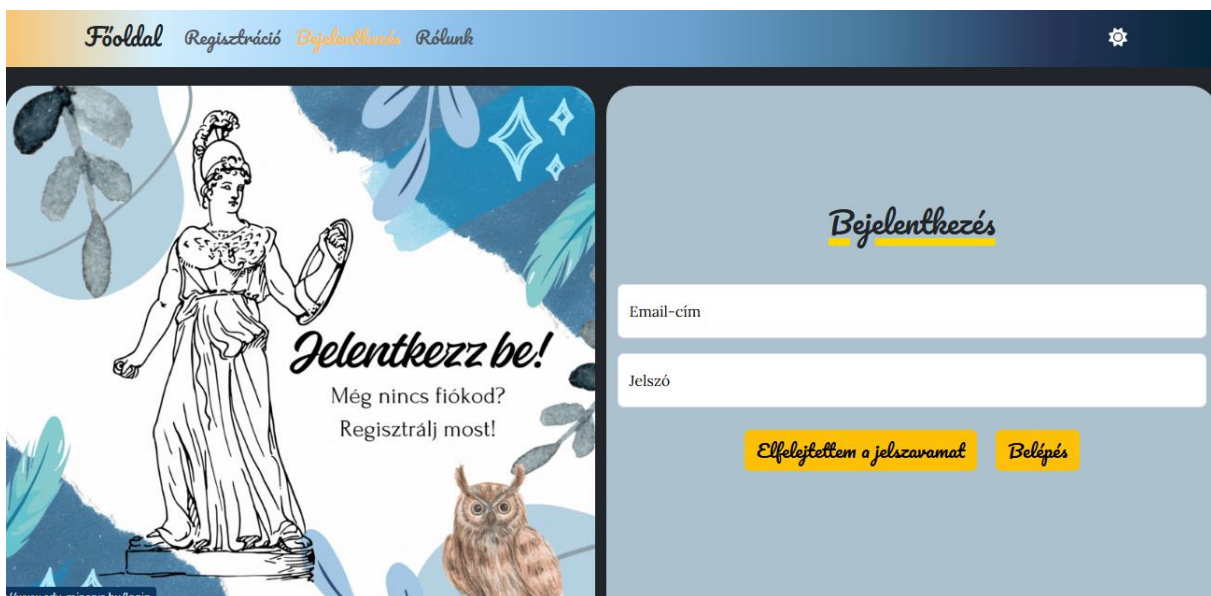
8. ábra: Bejelentkezés
