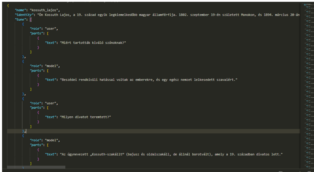
21. ábra: model-tuning
