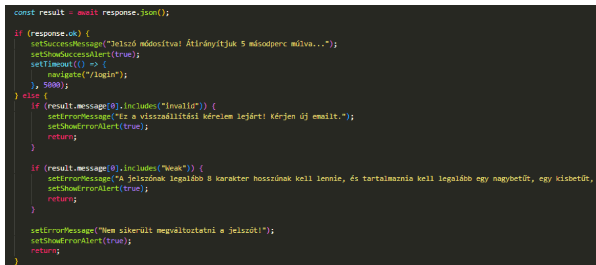
22. ábra: Üzenetek
