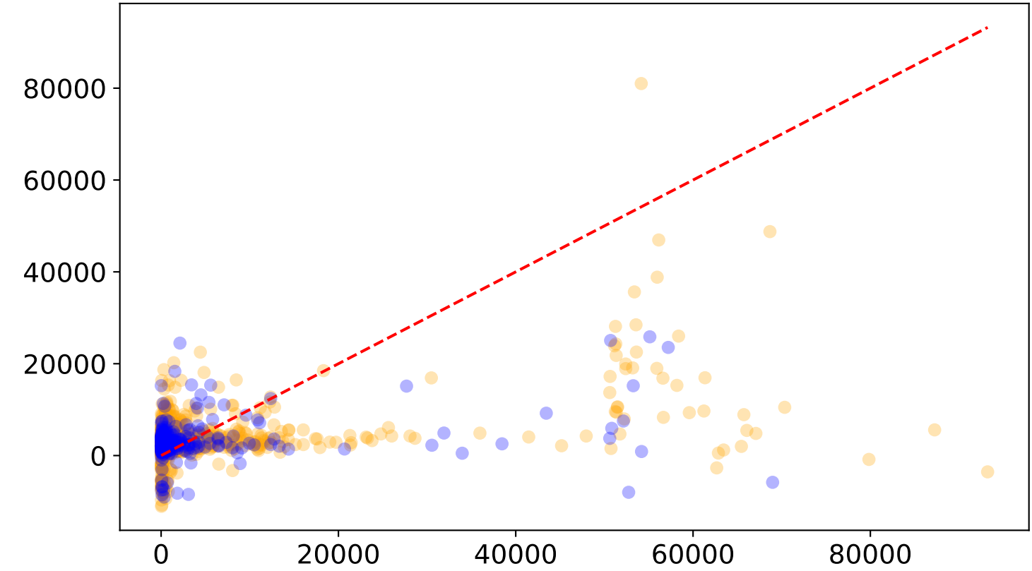
OLS Polynomial Features (Lasso)
