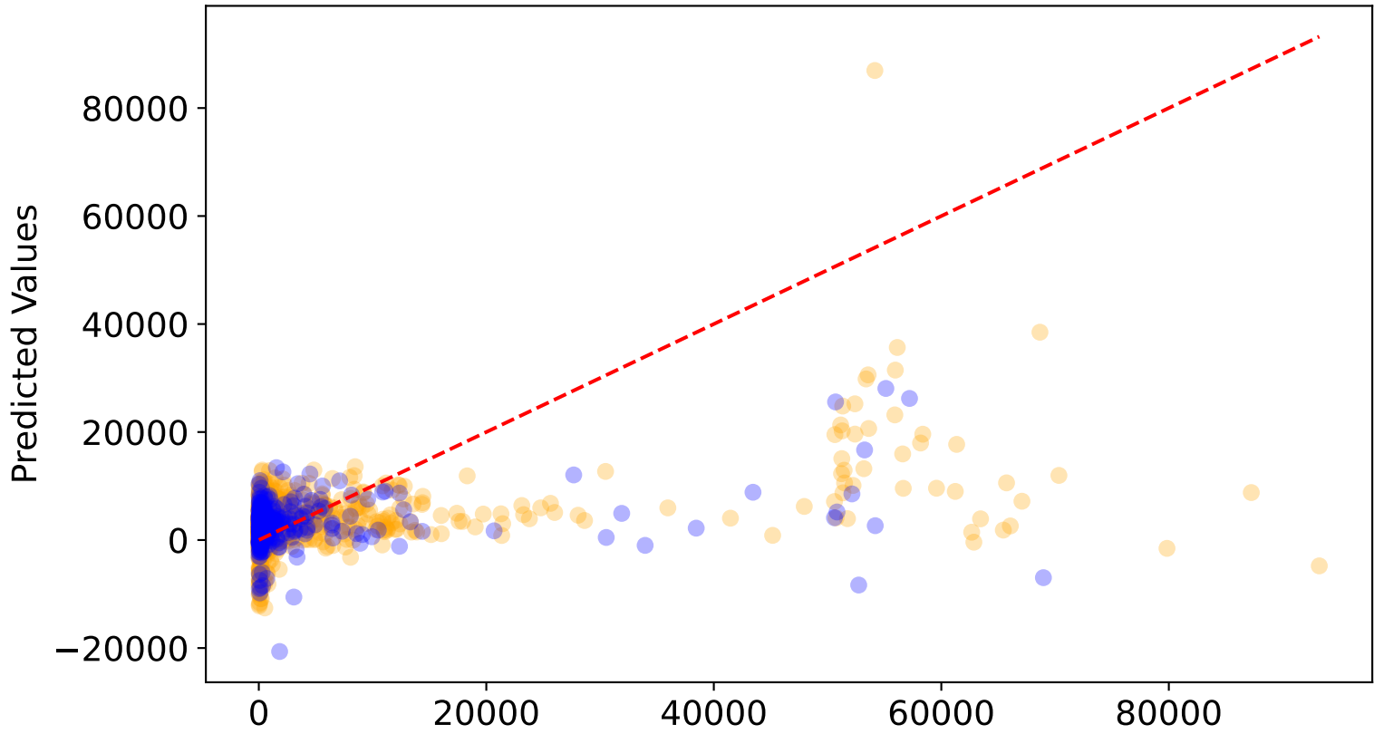
OLS (No Lasso)
