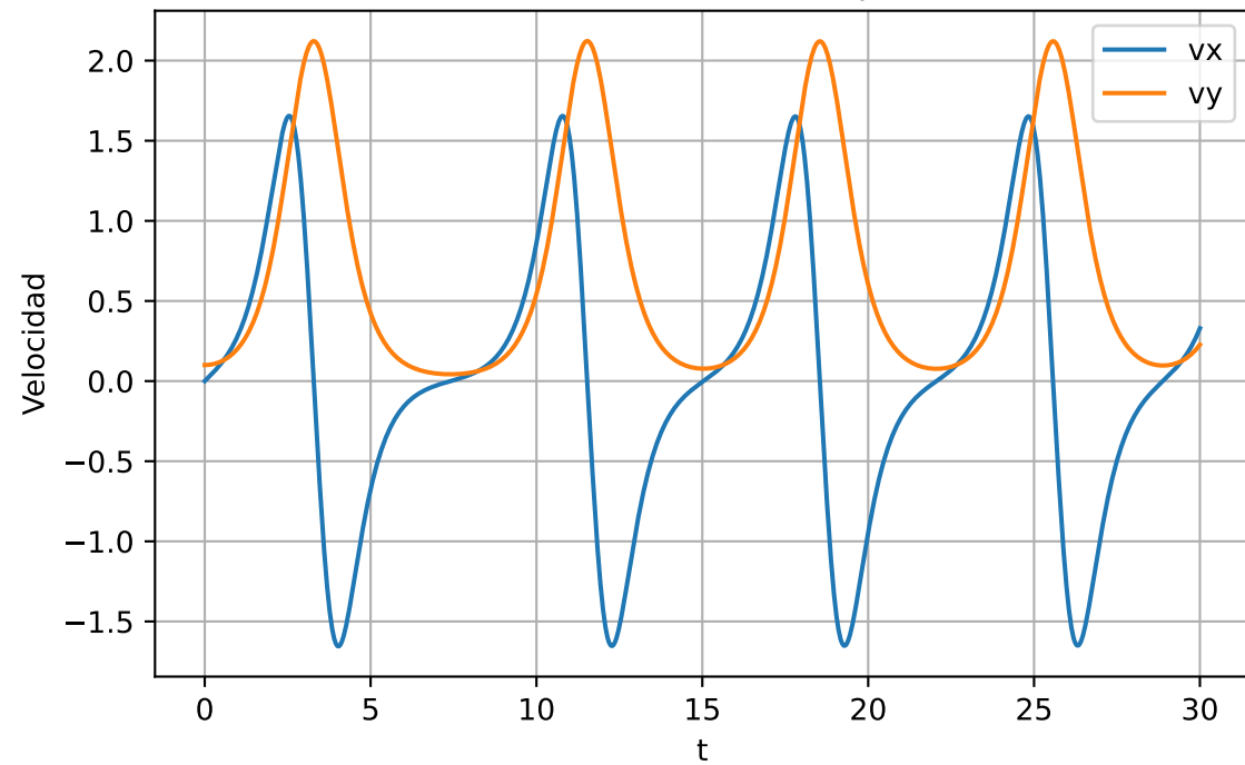
Velocidades vs tiempo
