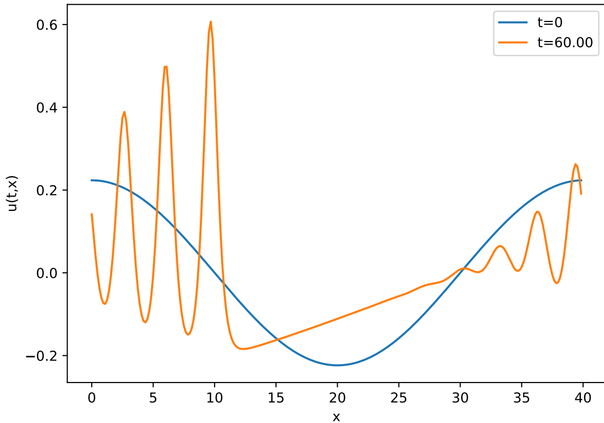
KdV (dif. finitas, periódicas)
