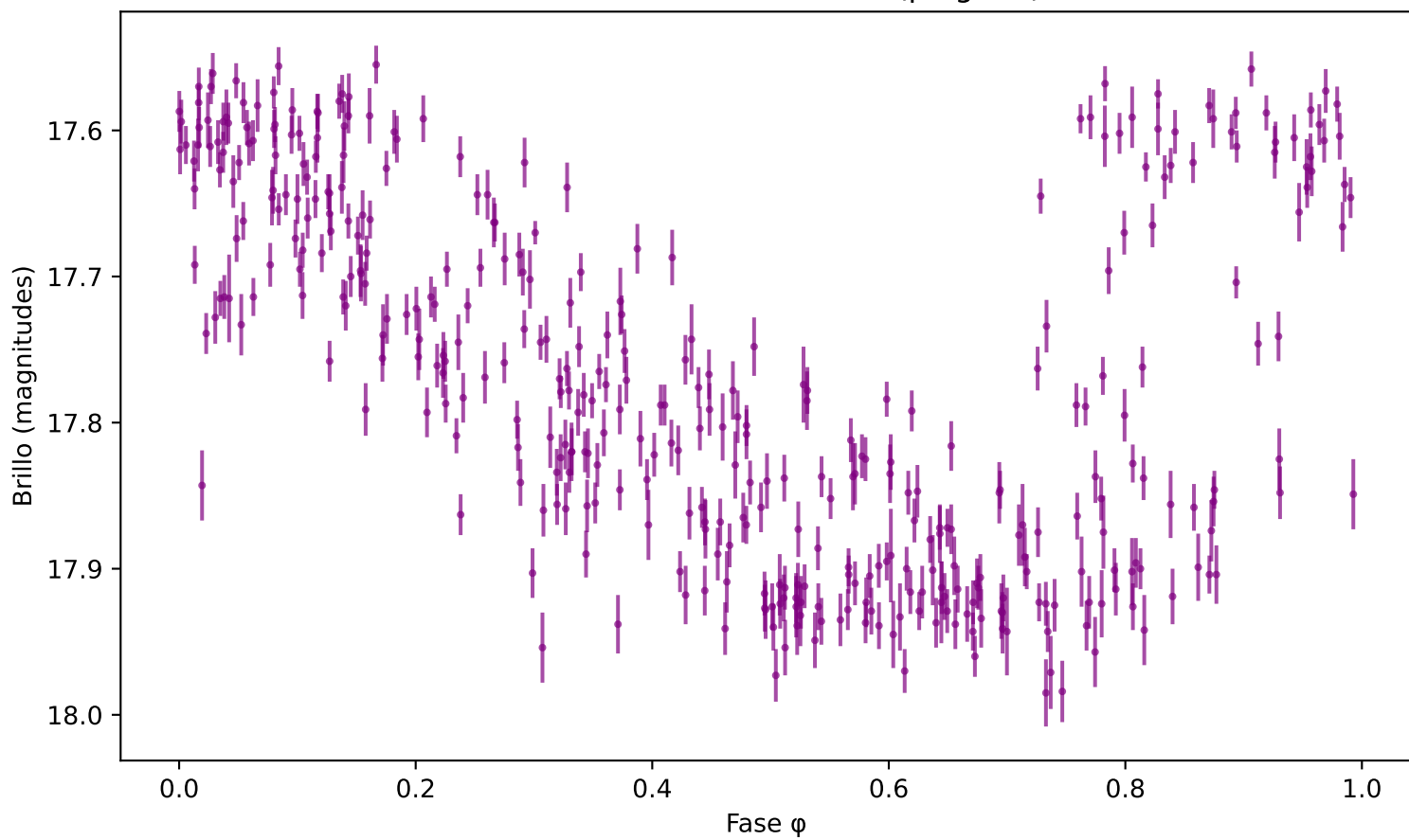
Curva de luz de la estrella (plegada)
