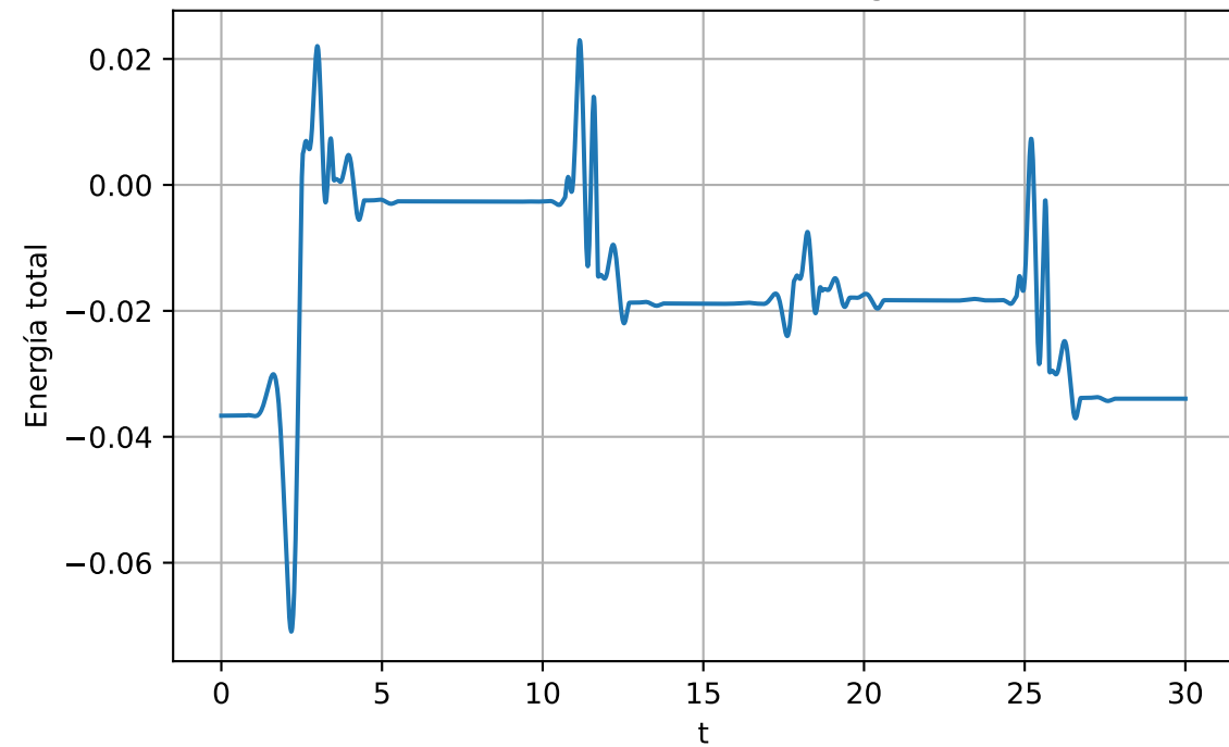
Conservación de energía
